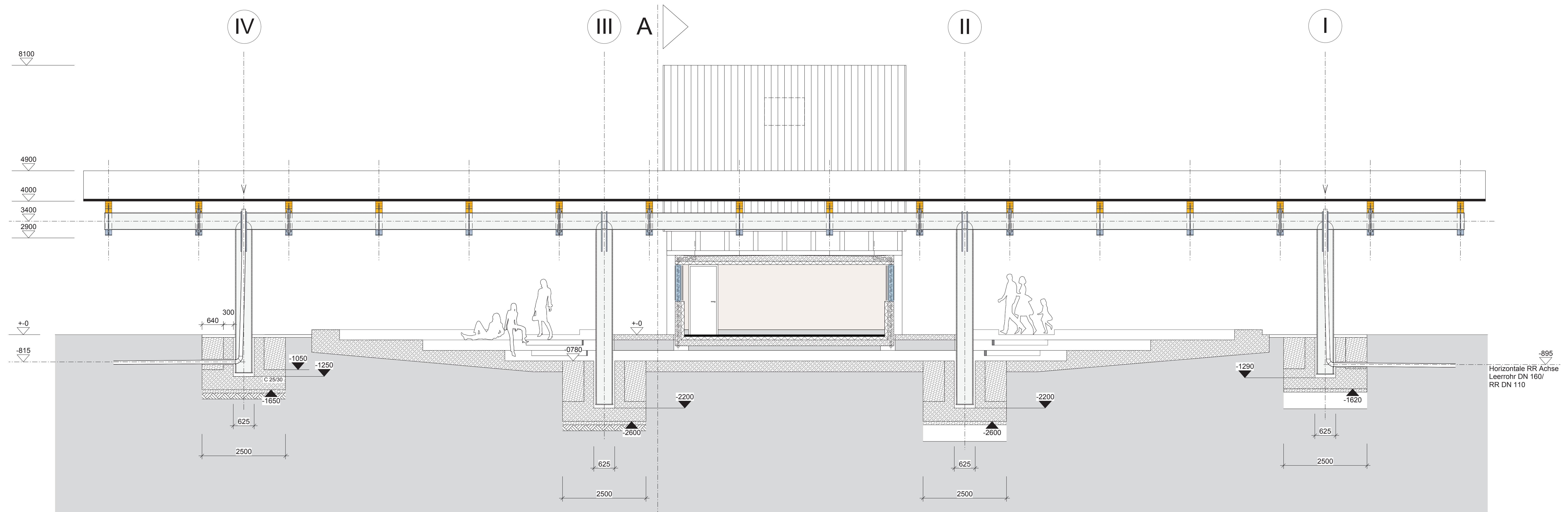
Schnitt B-B
