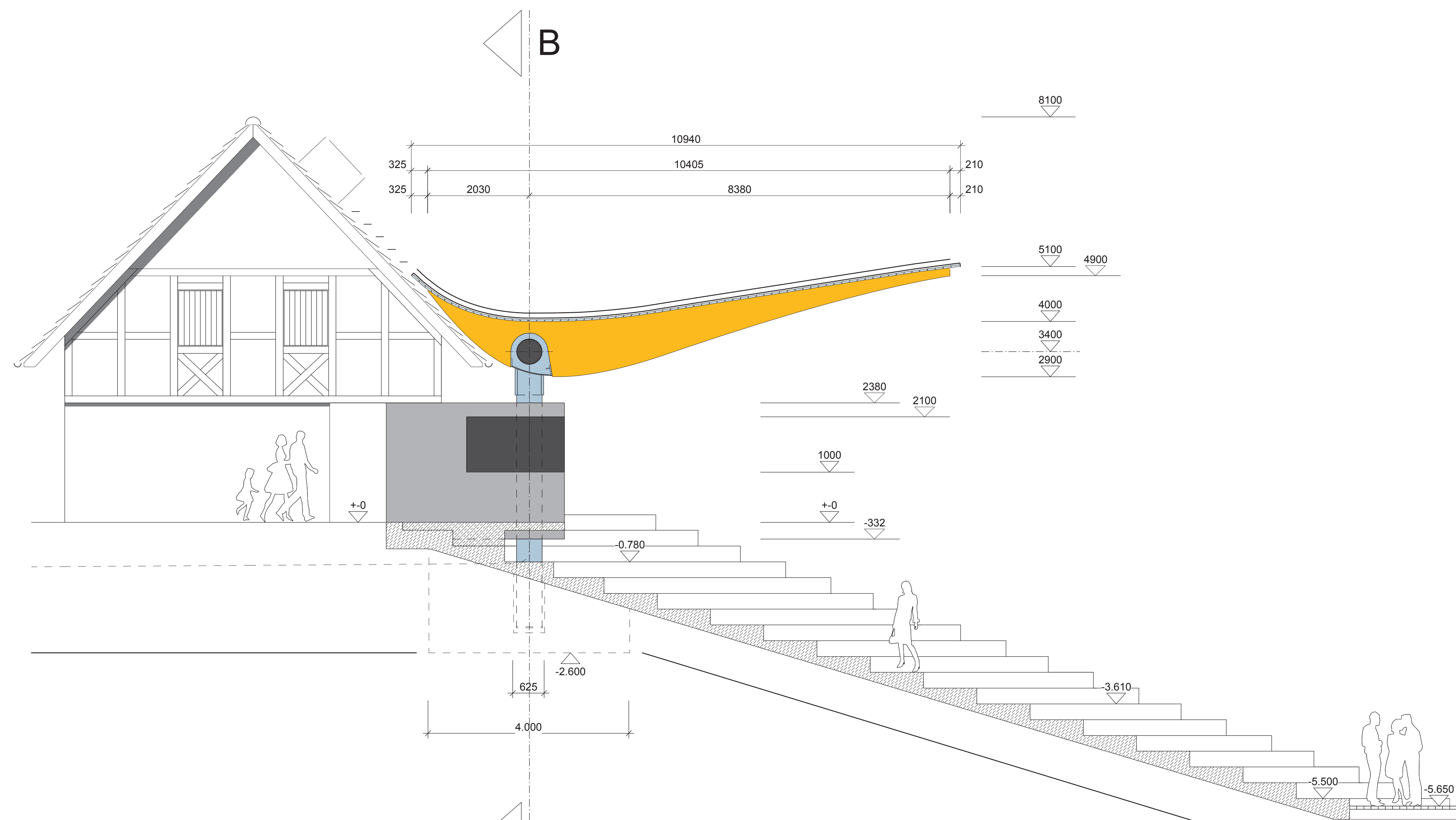
Schnitt A-A
