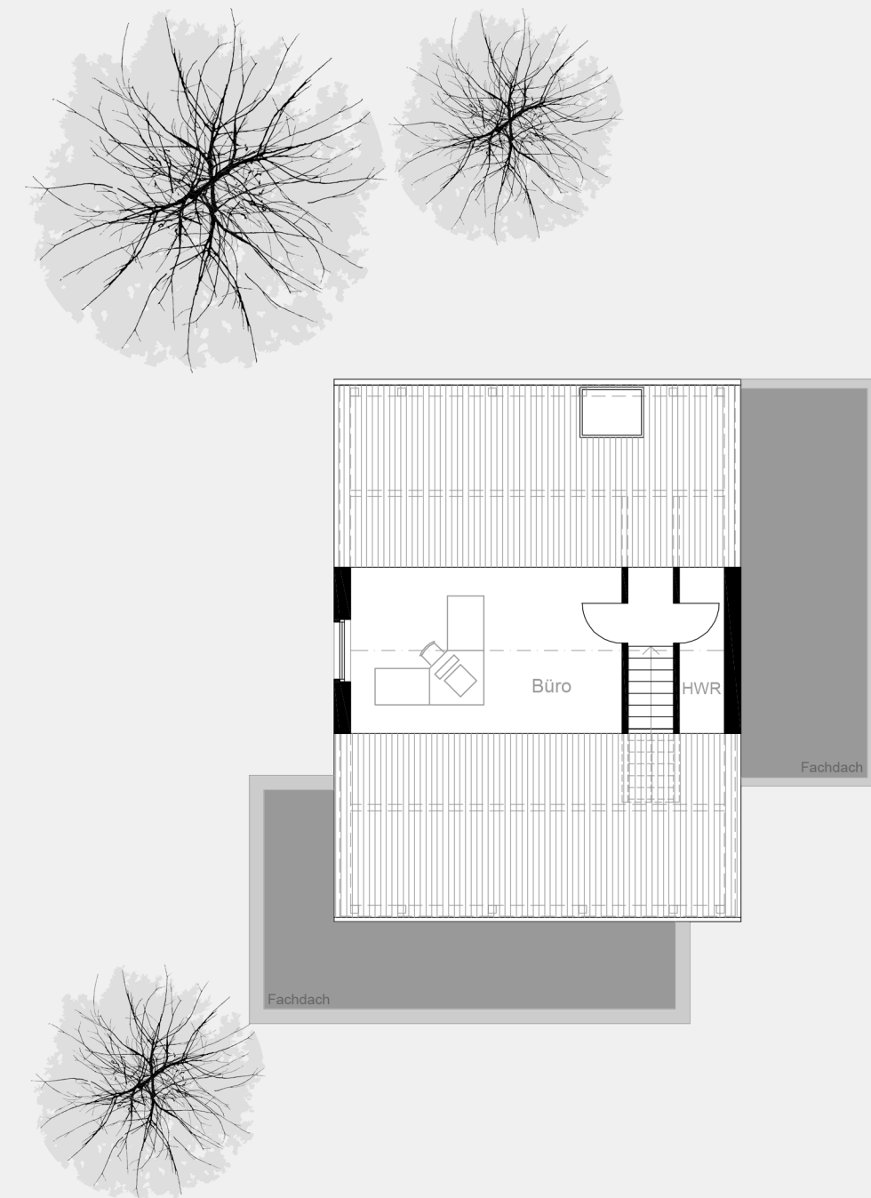
Grundriss Dachgeschoss
