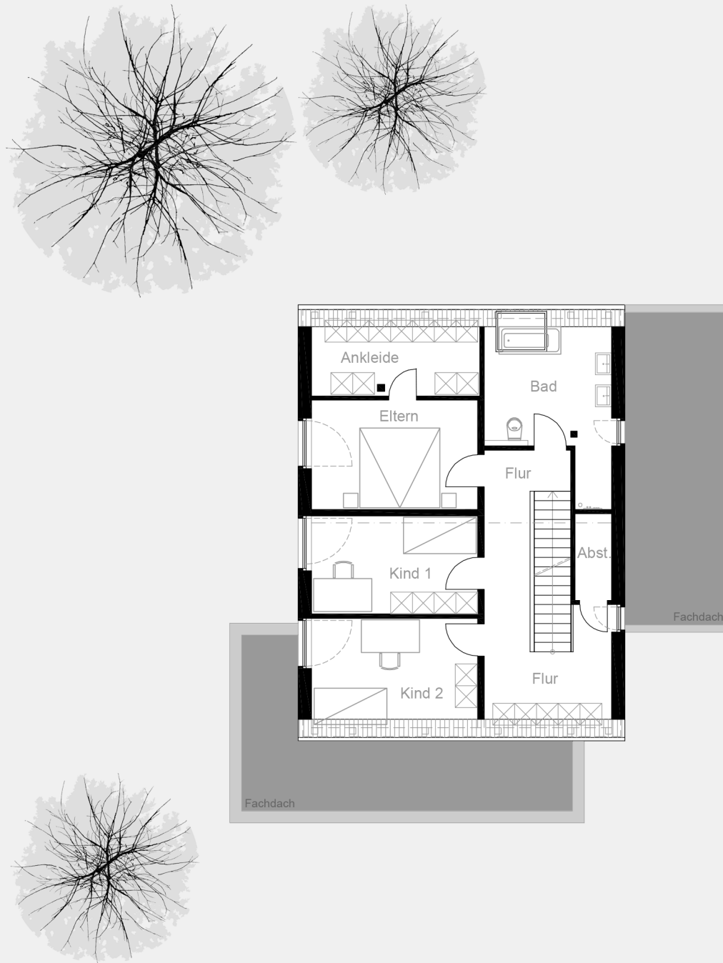
Grundriss Obergeschoss
