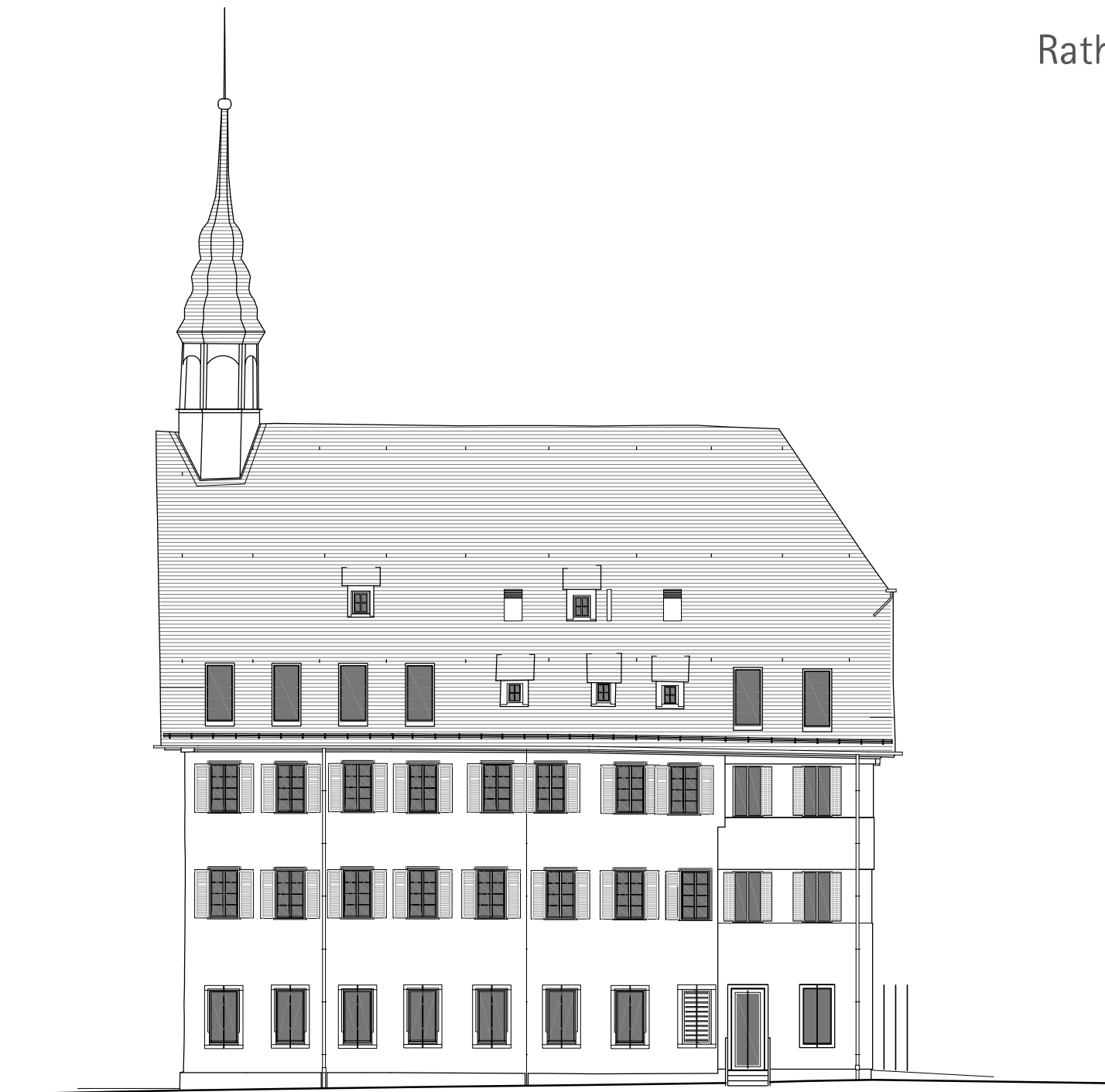
Ansicht Süd
