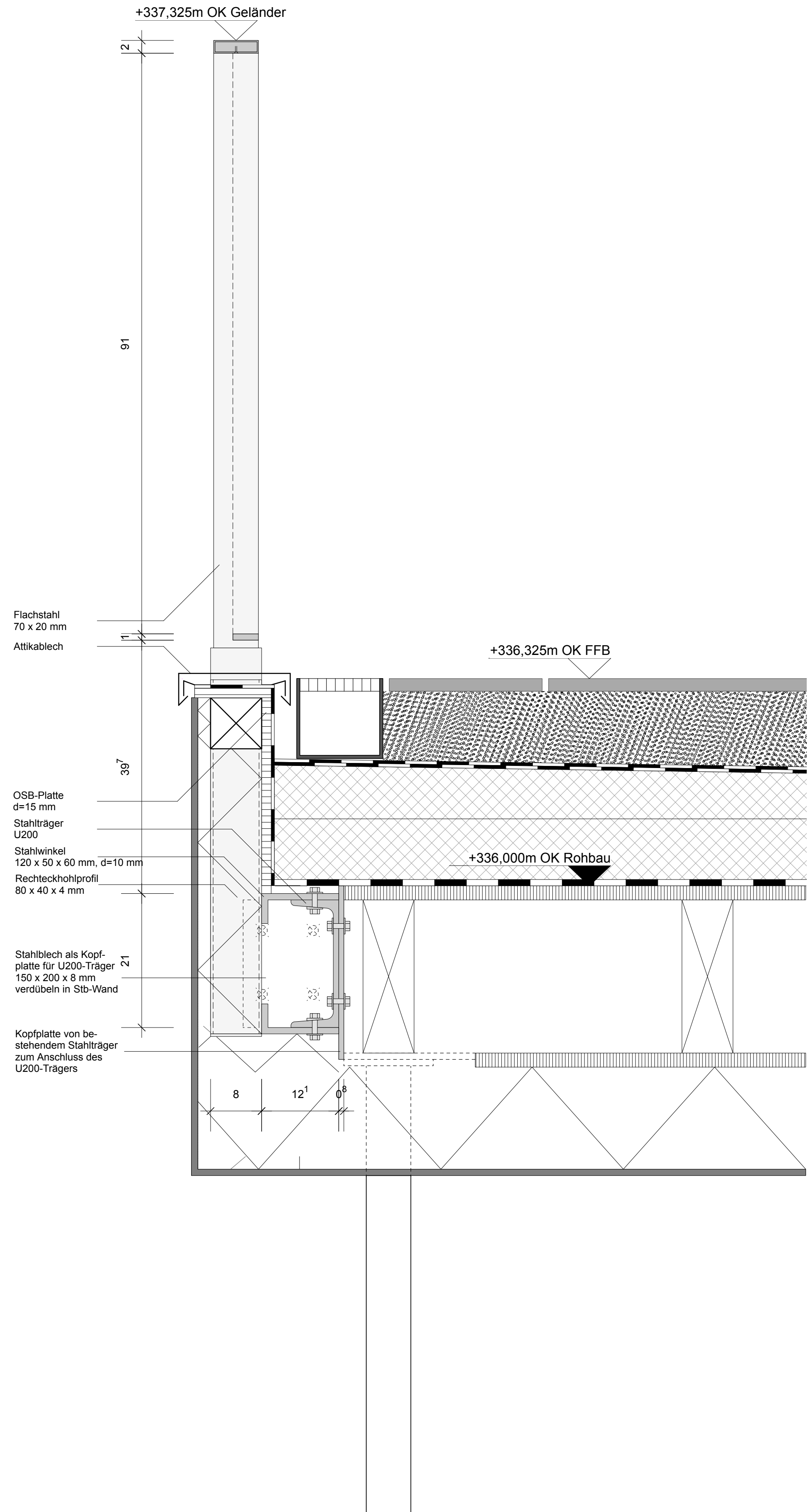
Detail 5 - Schnitt M1:5
