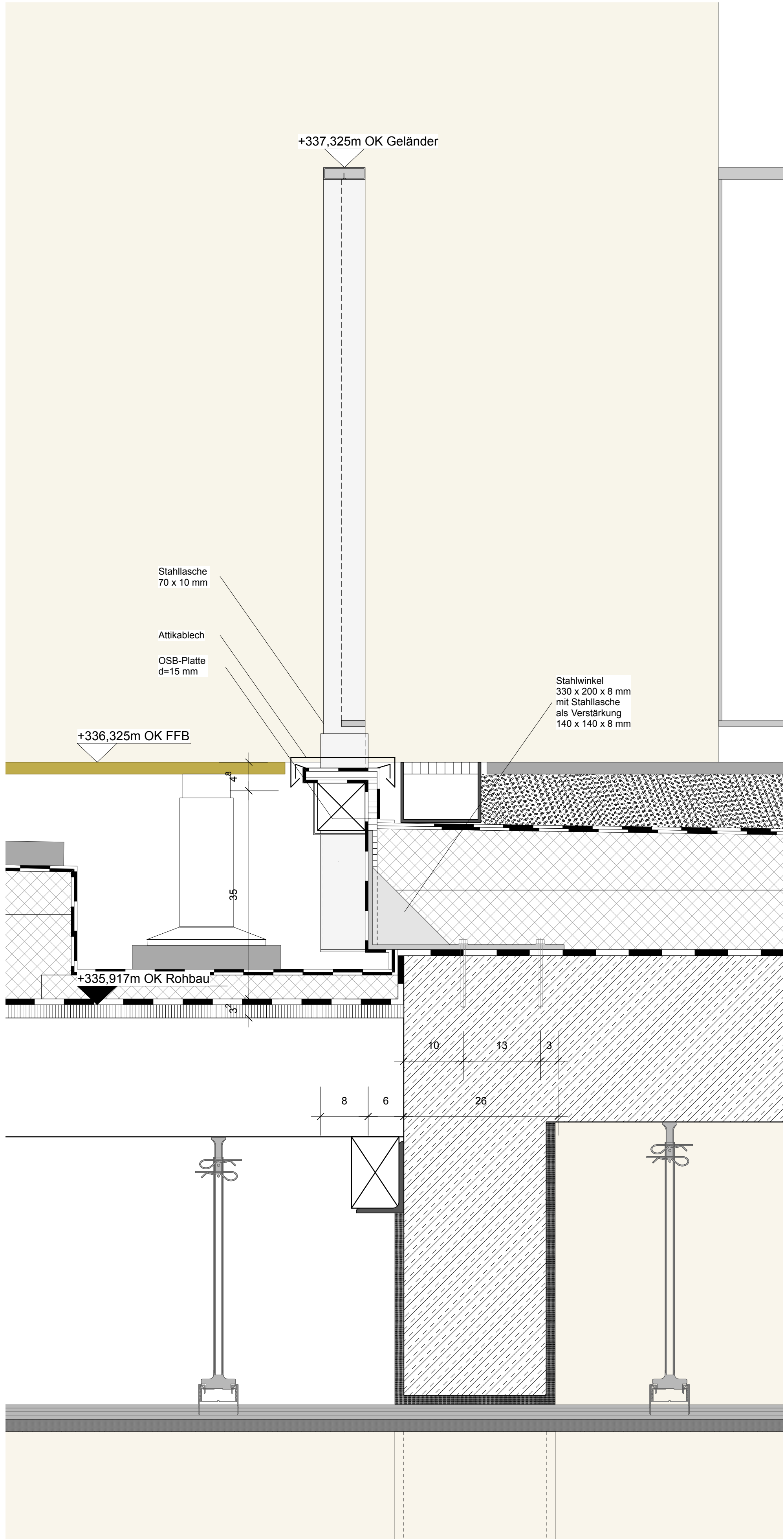
Detail 4 - Schnitt M1:5
