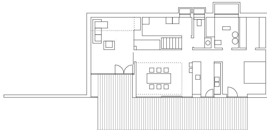
Grundriss Untergeschoss
