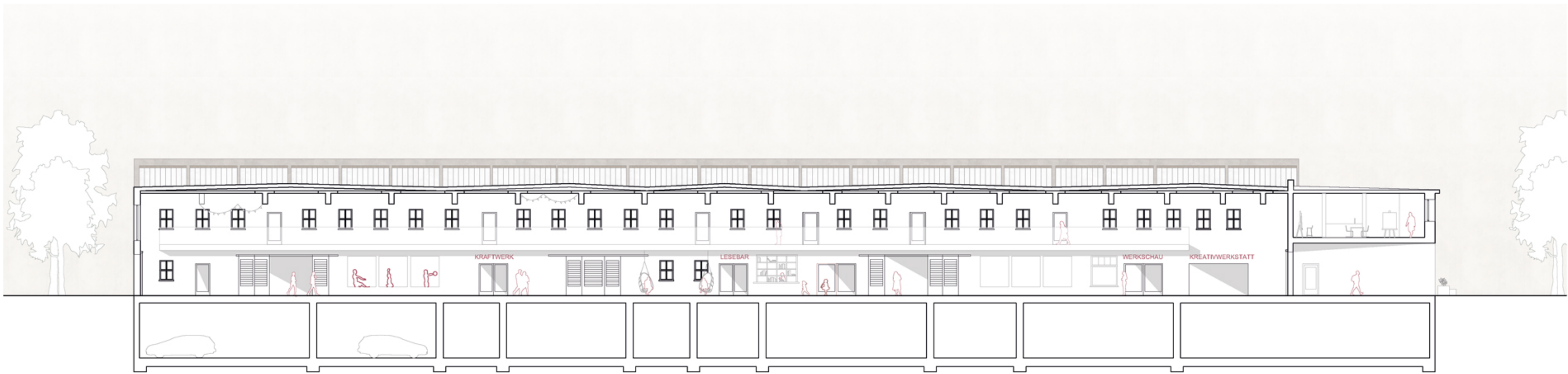
Schnitt C-C M 1:200
