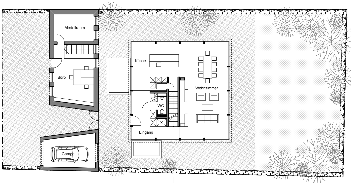
ERDGESCHOSS
