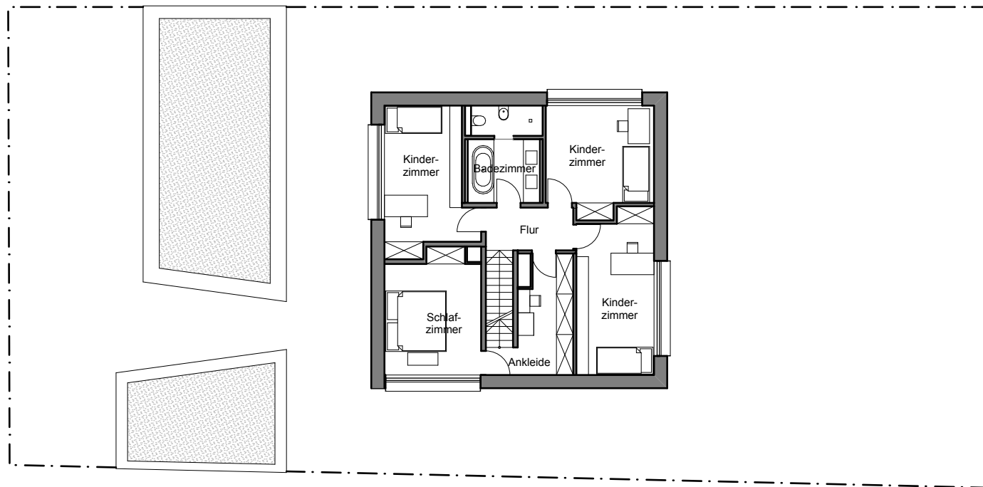
OBERGESCHOSS
