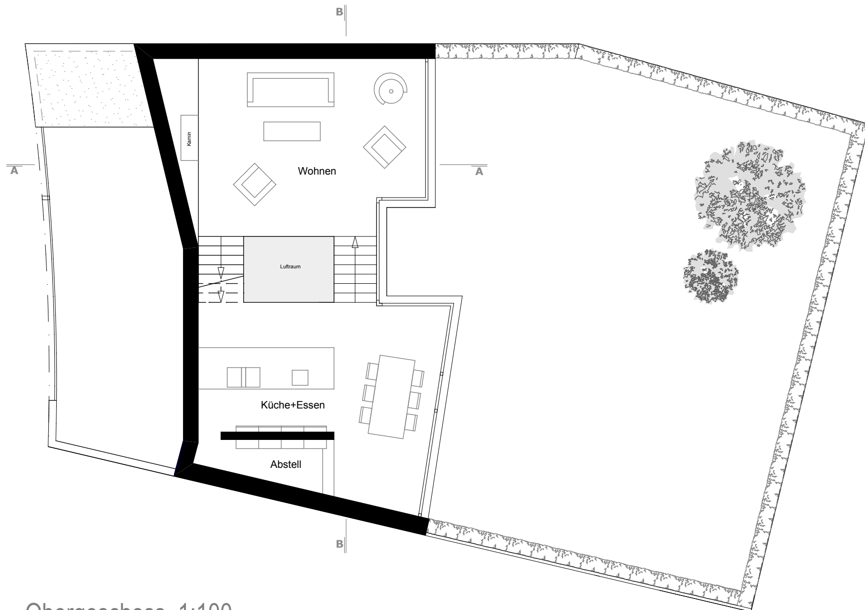
Obergeschoss 1:100
