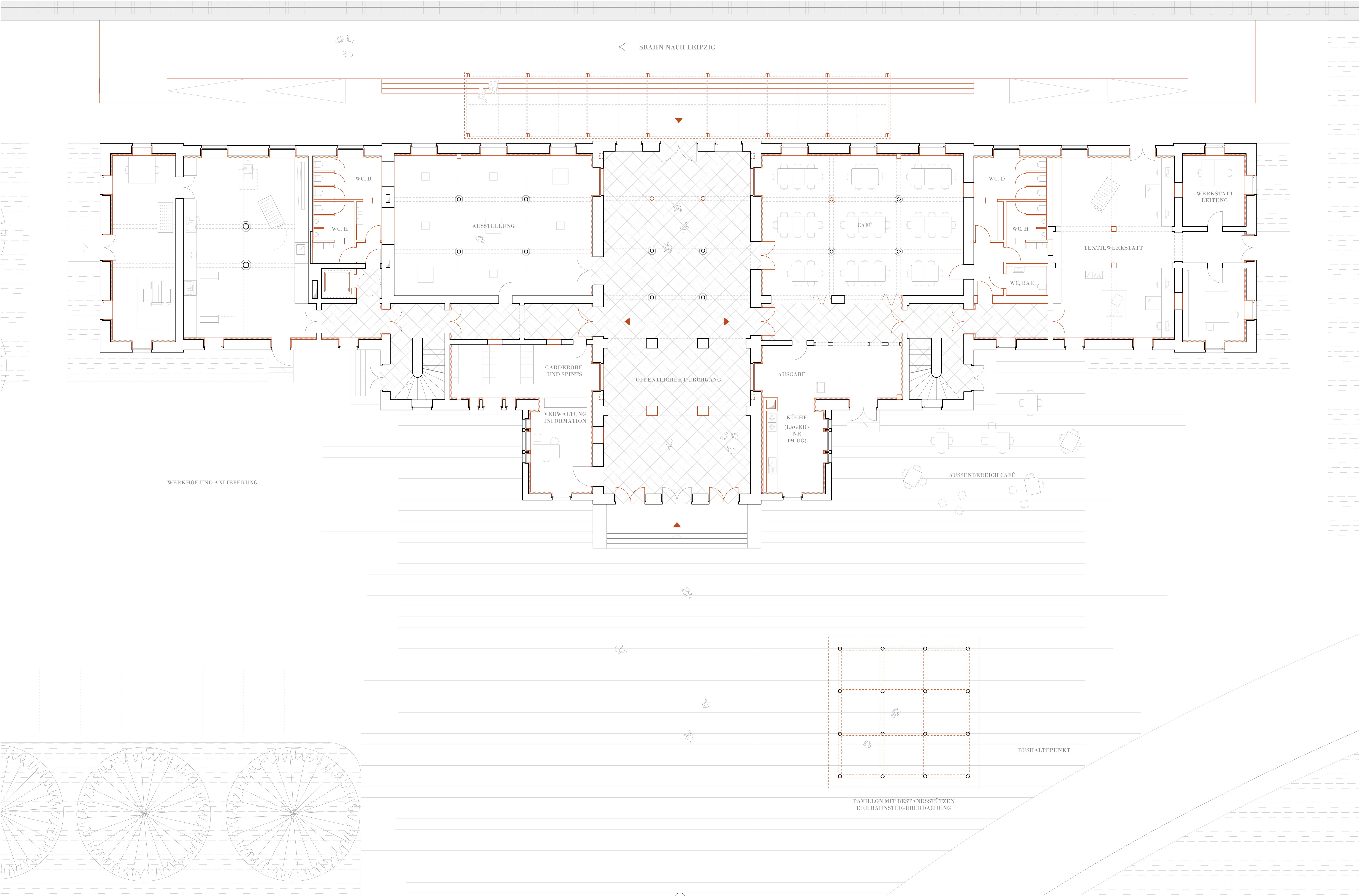
ERDGESCHOSS 1:100
