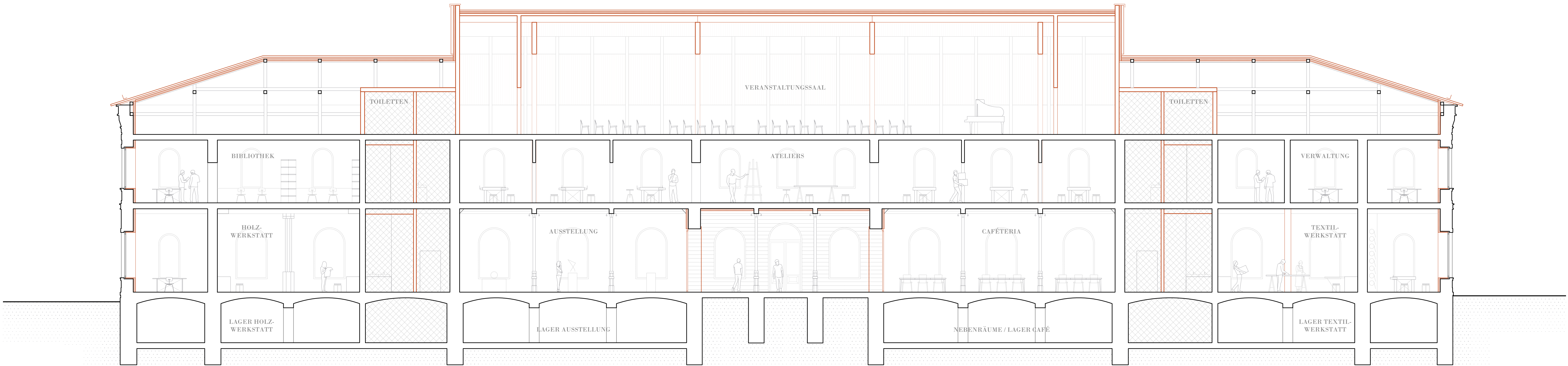
LÄNGSSCHNITT 1:100
