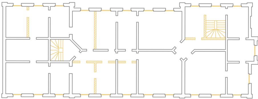
1.OG
