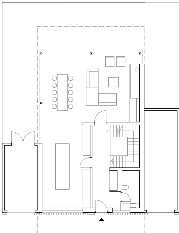
Erdgeschoß
