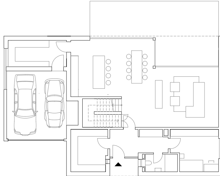
Erdgeschoß
