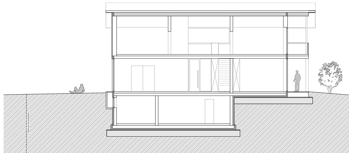
Querschnitt
