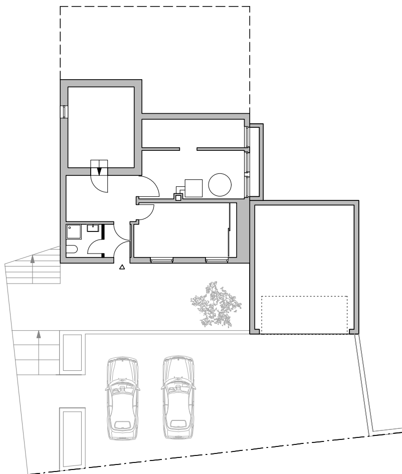
GRUNDRISS UG 1:200
