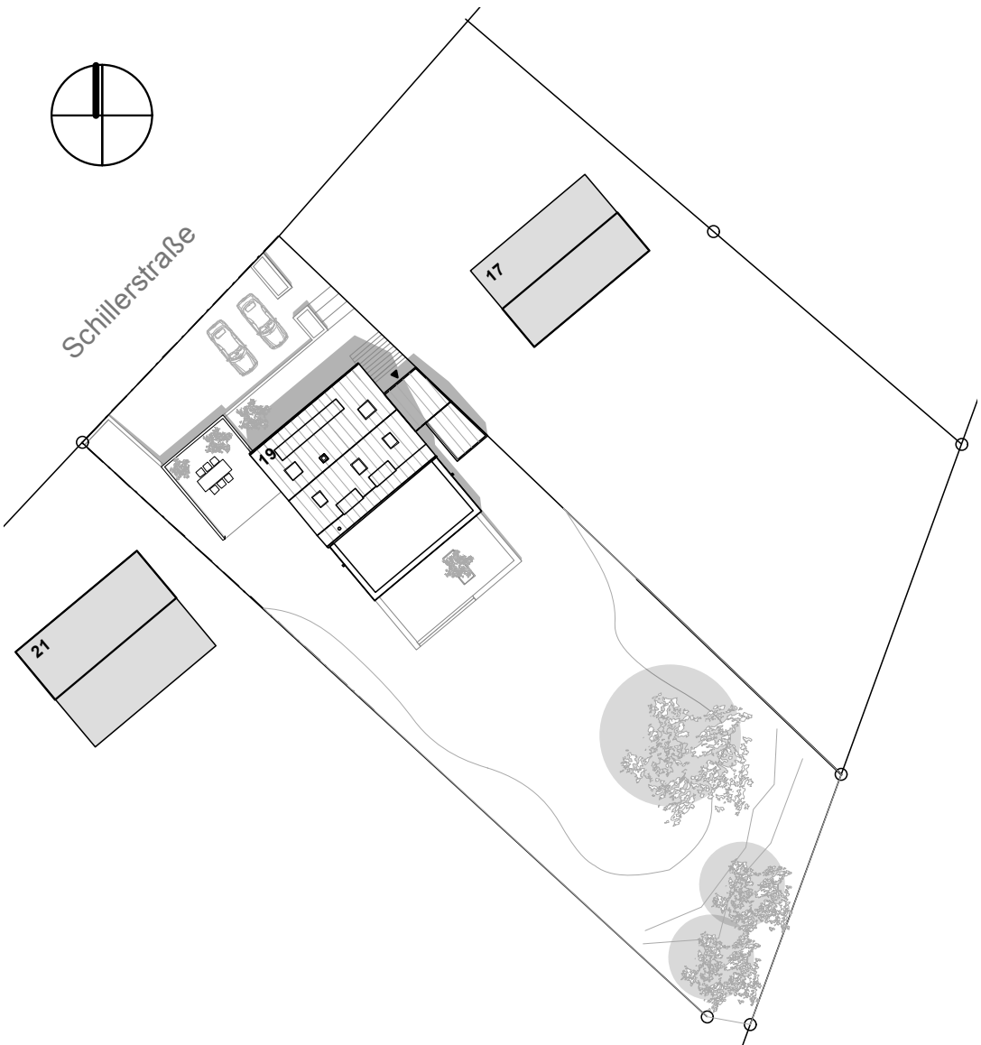
LAGEPLAN 1:500
