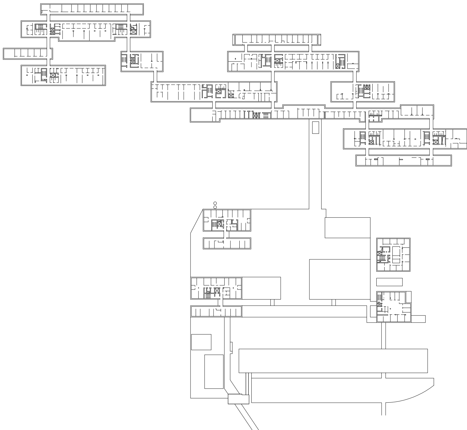
Riegler Riewe Architekten / Med Uni Campus Graz / 4 Obergeschoss / Level 4
