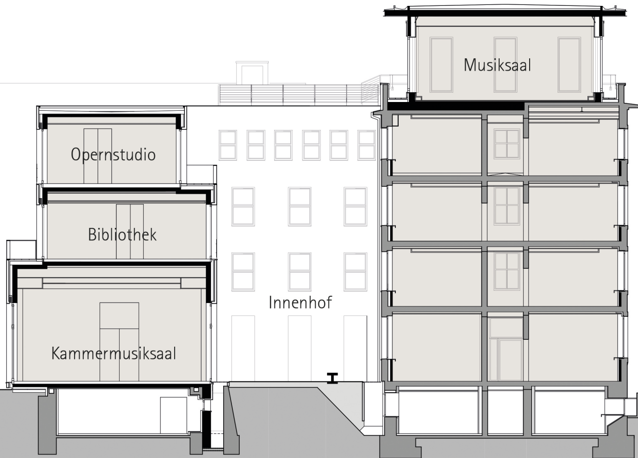
Schnitt 1-1, Ostansicht Innenhof
