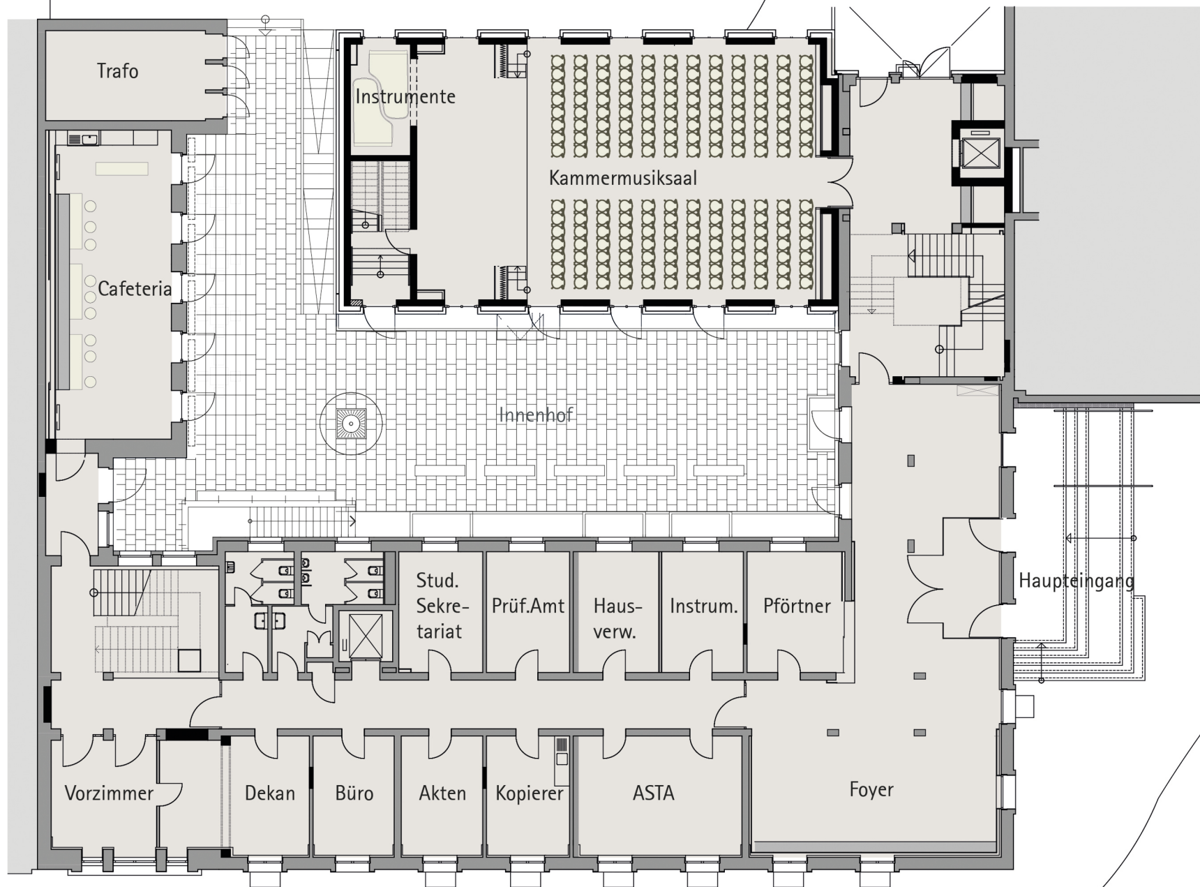
Grundriss EG
