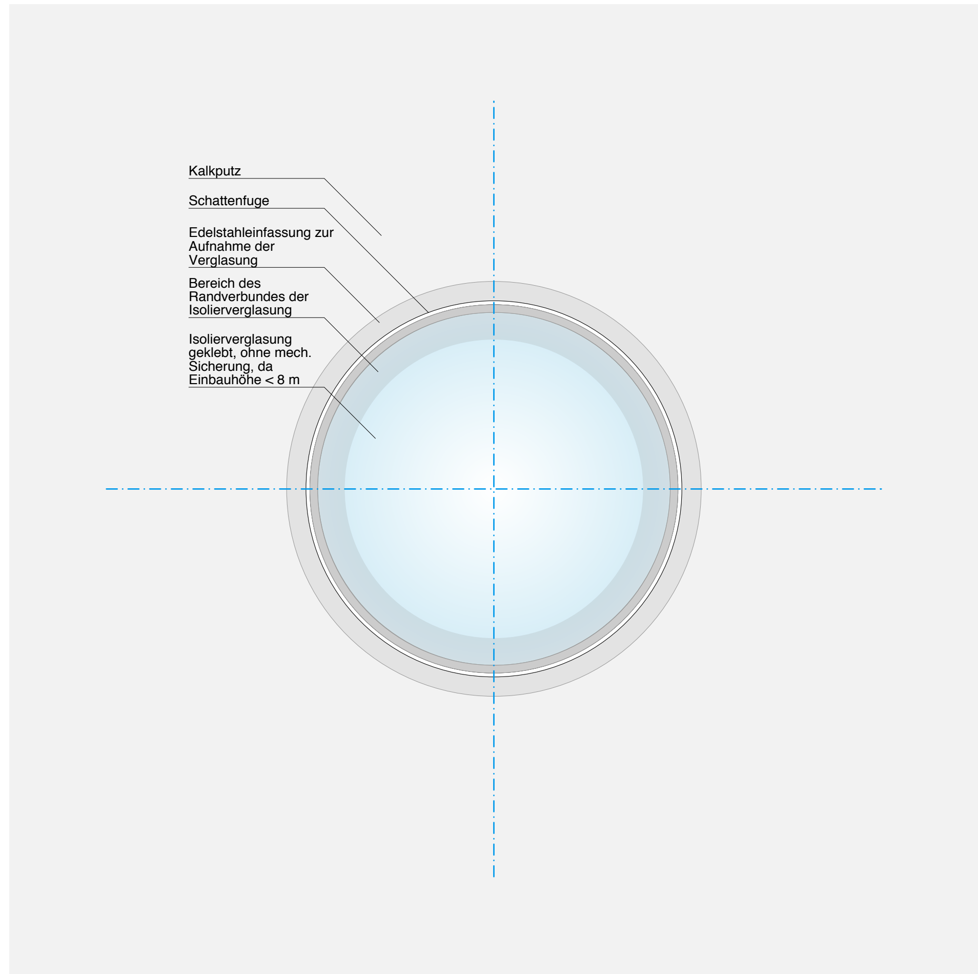
Aussenansicht
