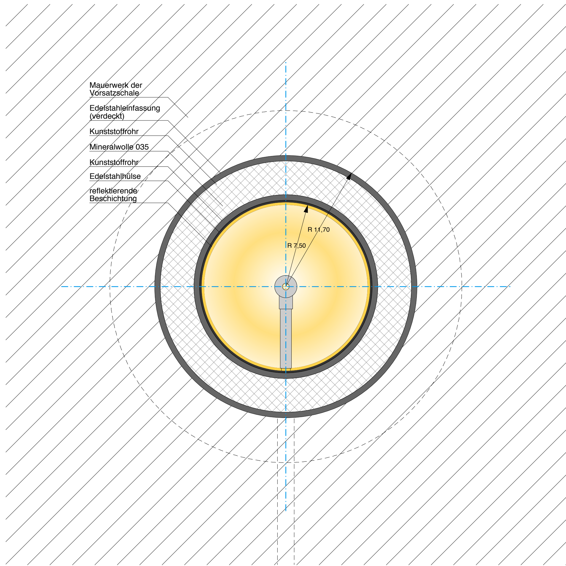
Schnitt Quer
