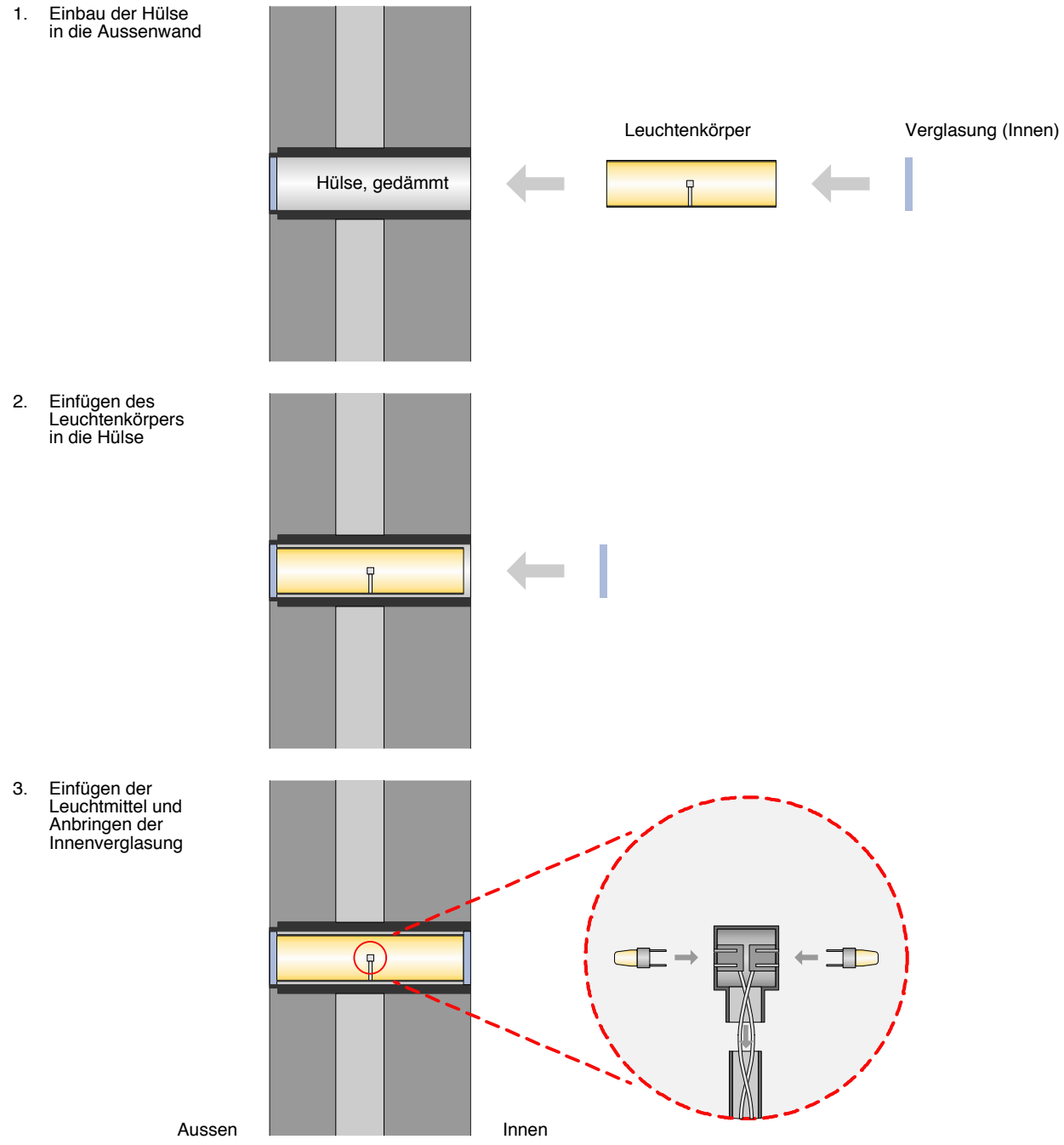
Schnitt Längs
