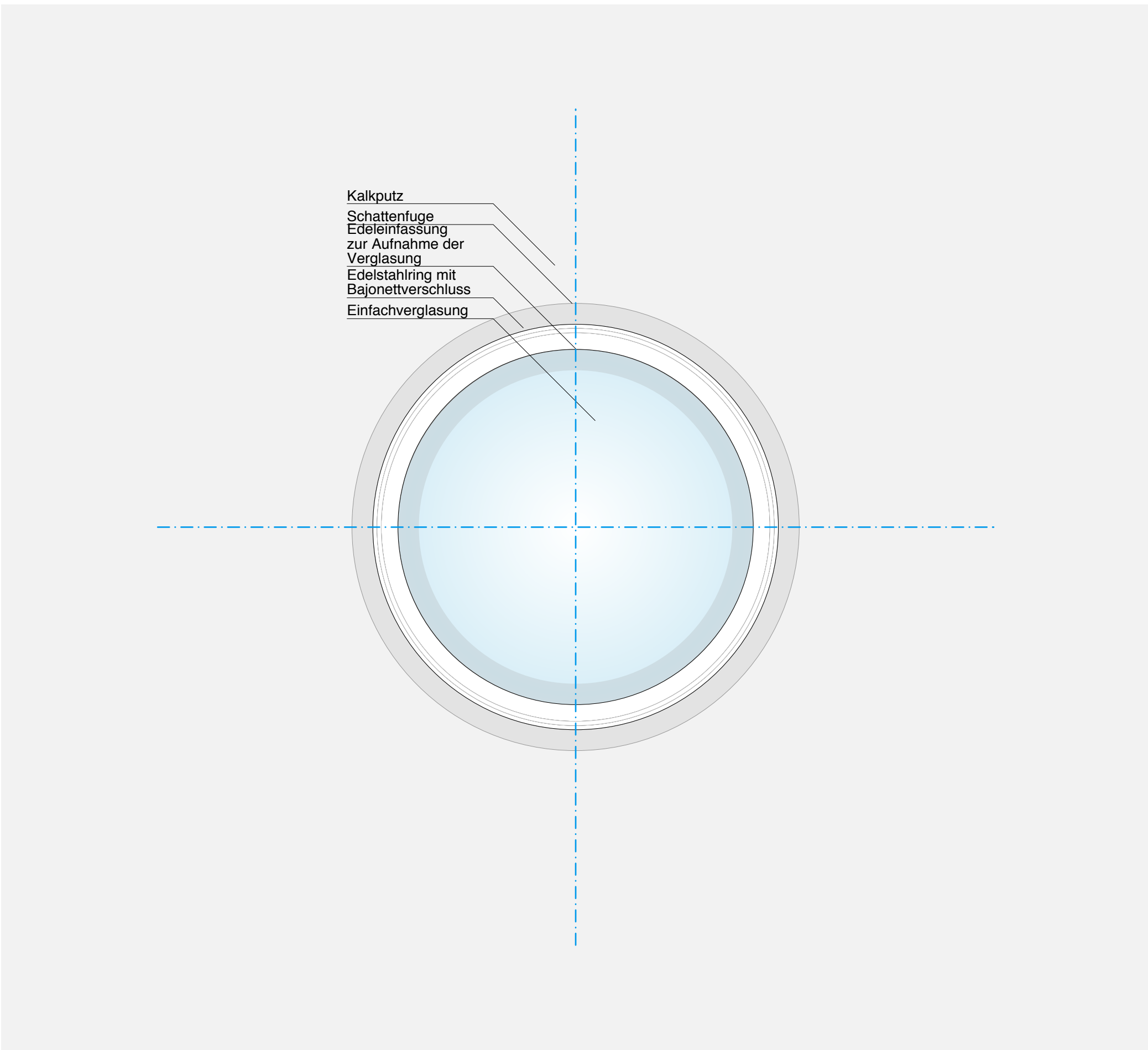
Innenansicht
