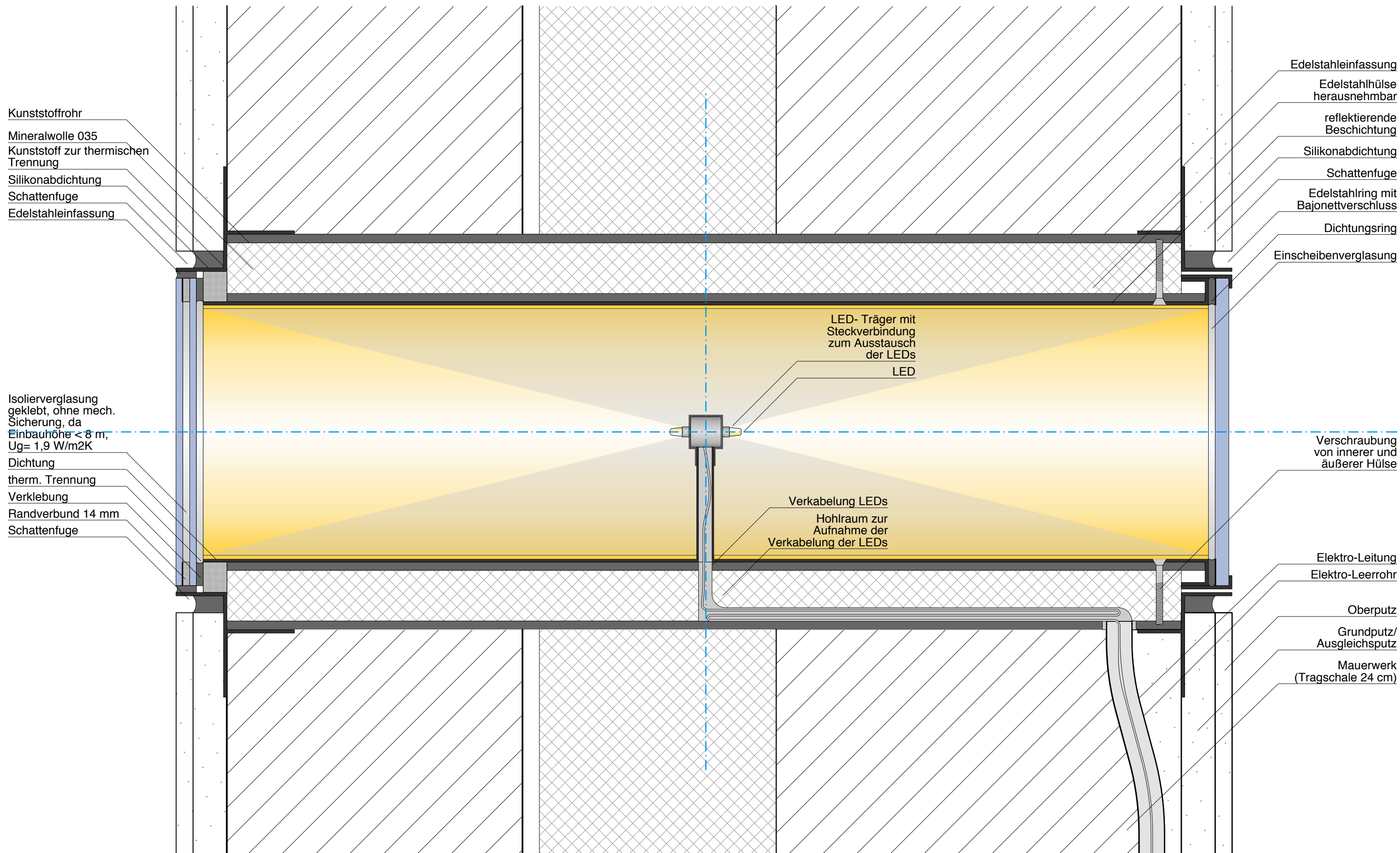
Schnitt Längs
