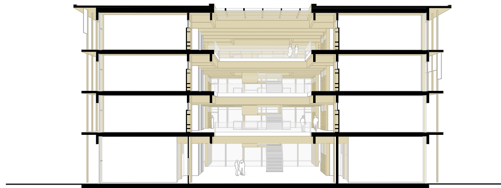
Querschnitt Galerien
