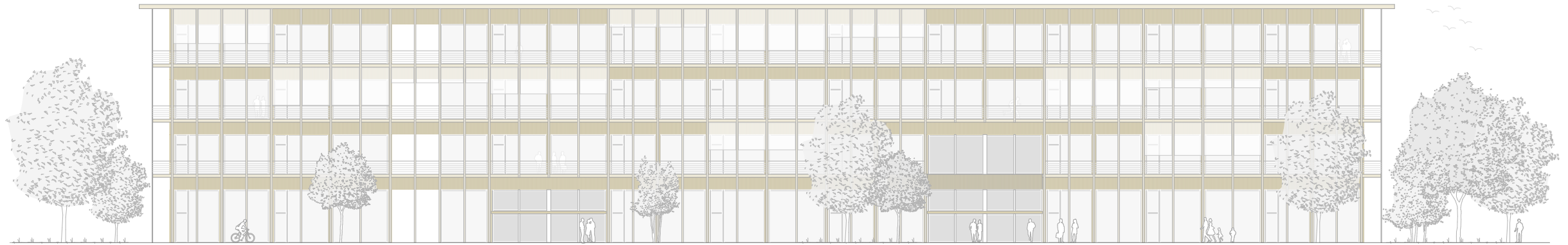
Ost Ansicht
