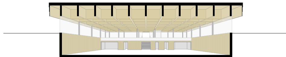
Querschnitt
