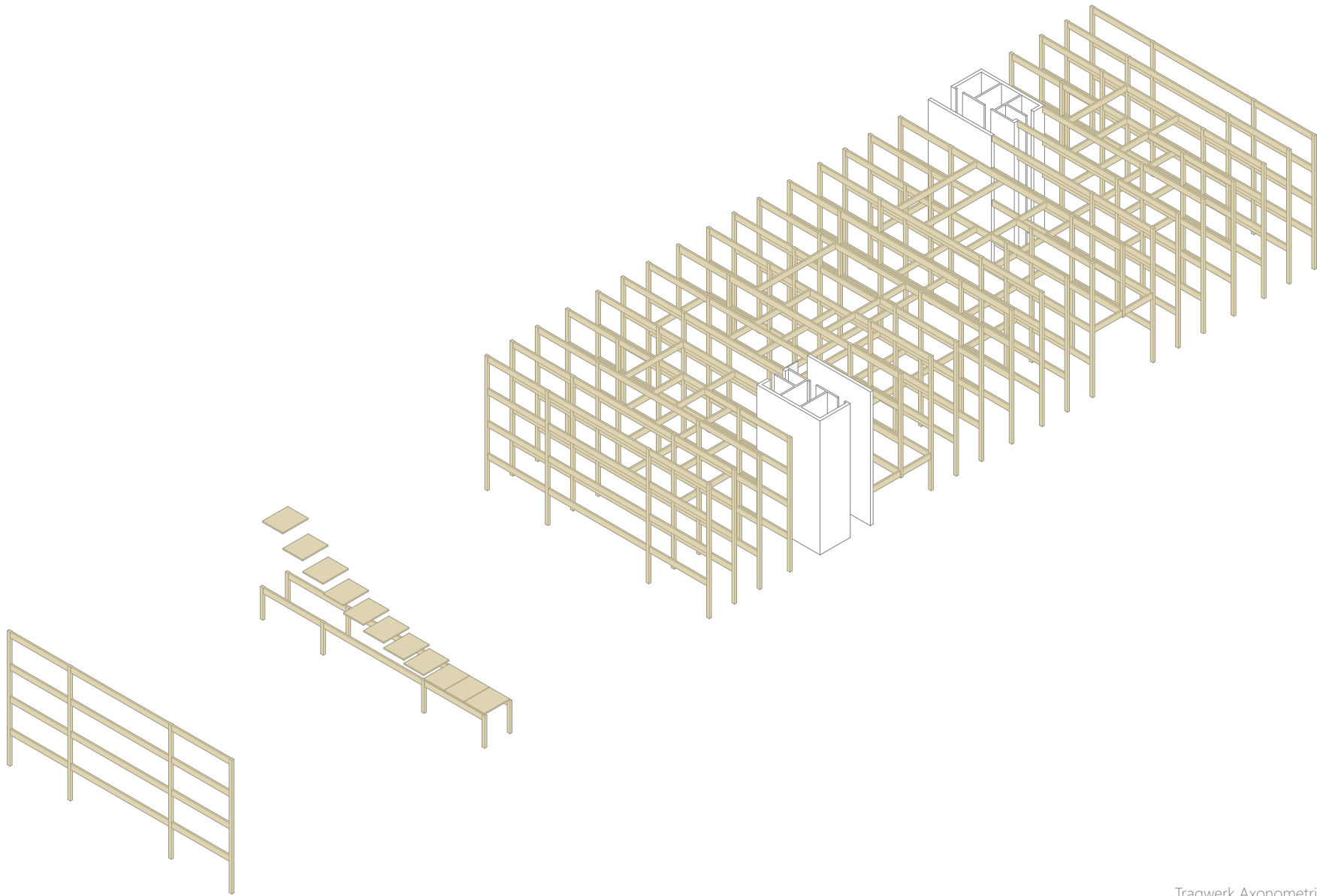
Tragwerk Axonometrie
