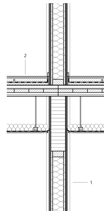
Detail - Querschnitt 1:20
