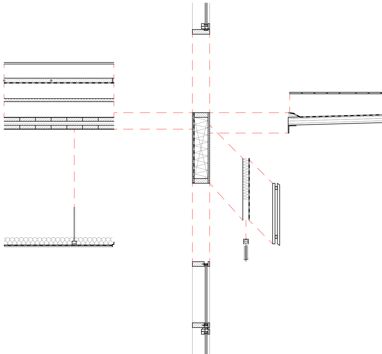
Detailschnitt - Vorfertigung
