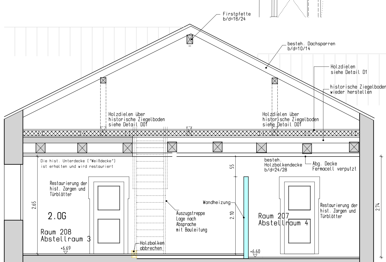
Schnitt F-F
