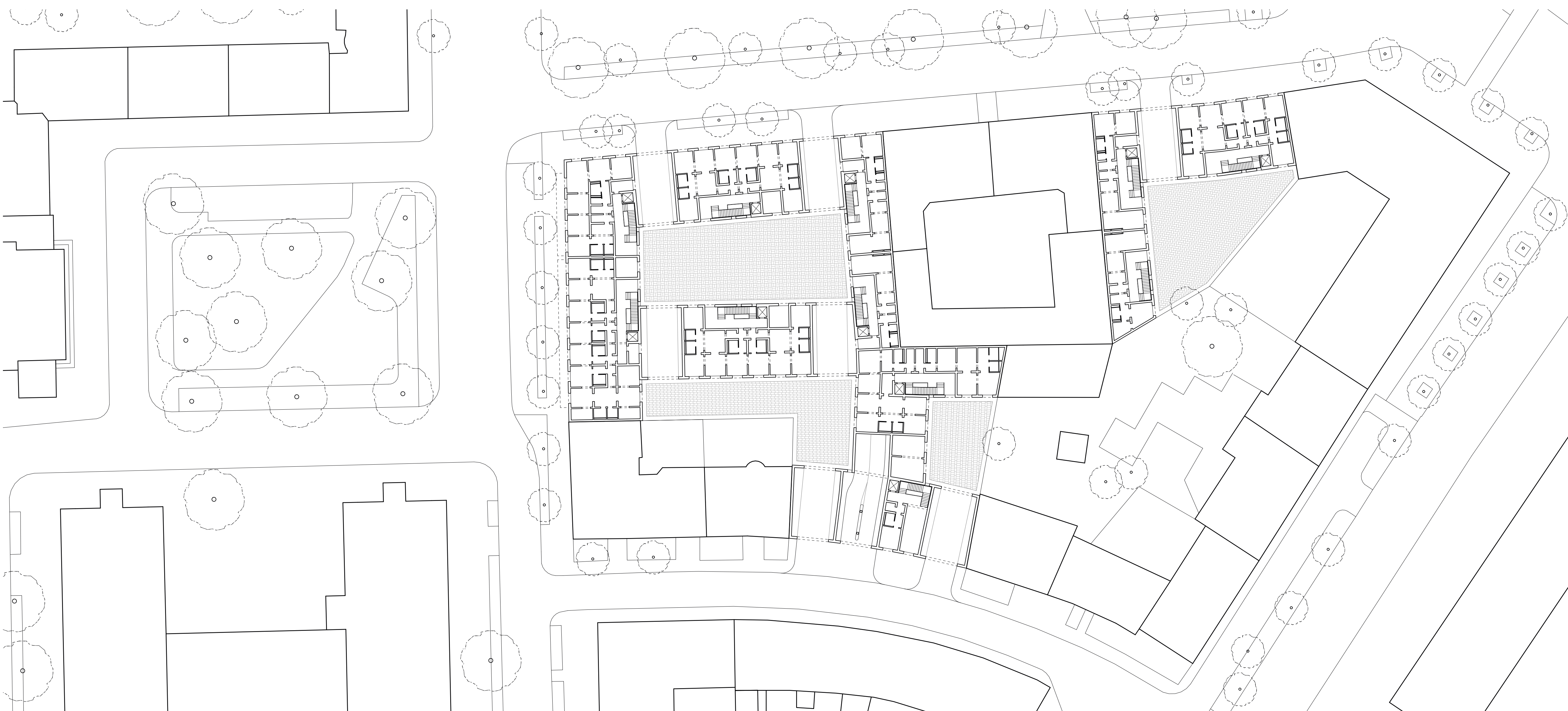
Grundriss Erdgeschoss M 1:400
