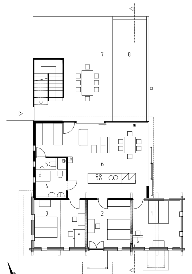
Grundriss Erdgeschoß
