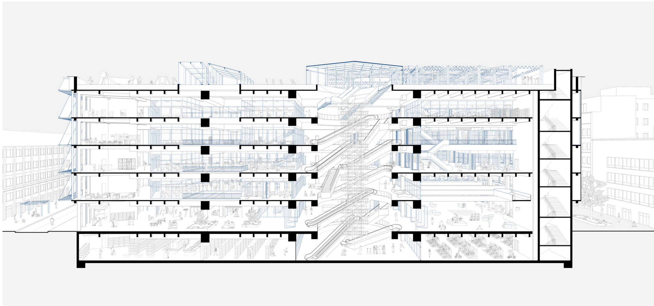
Perspektivischer Schnitt
