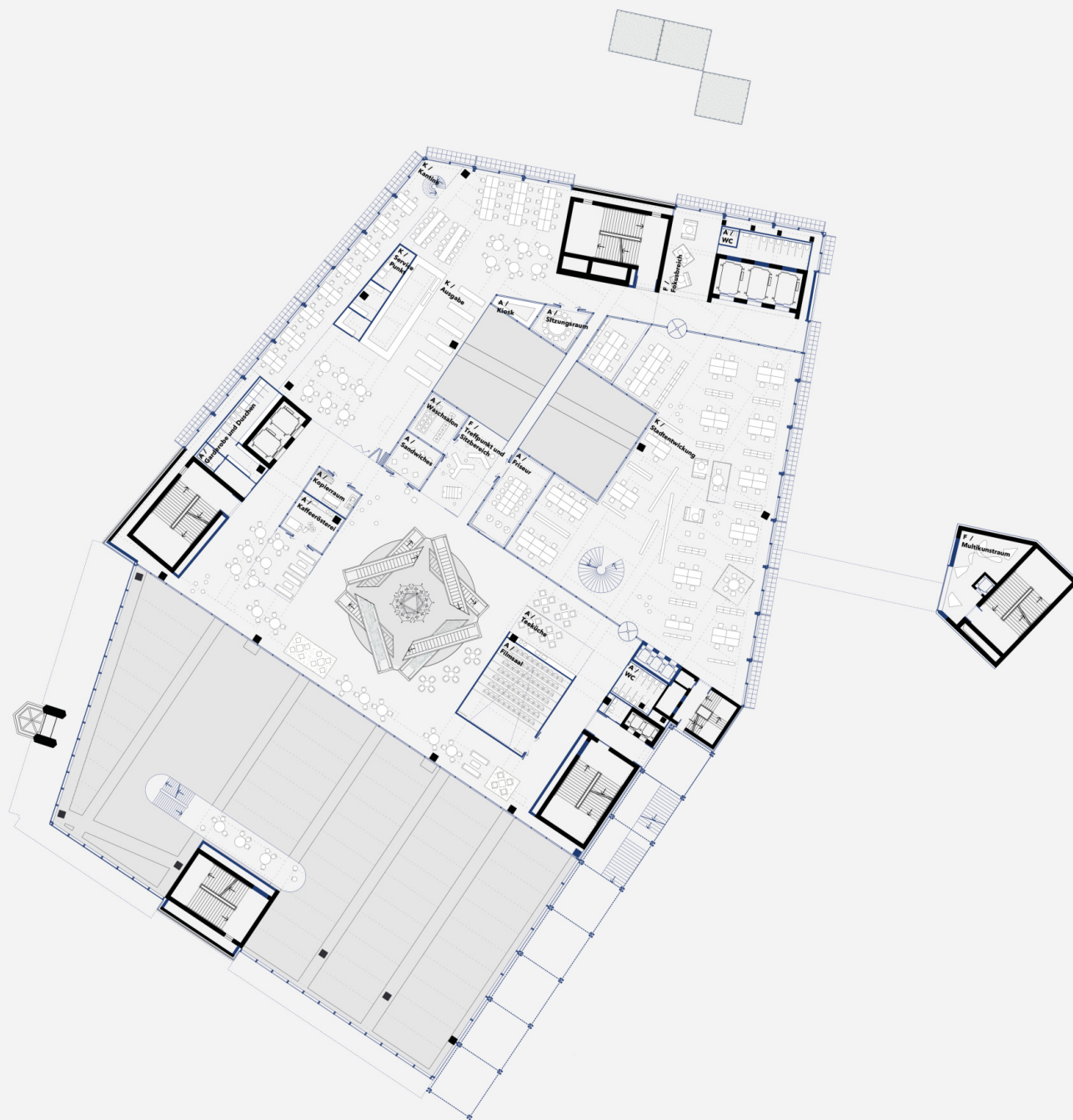
Obergeschoss 01
