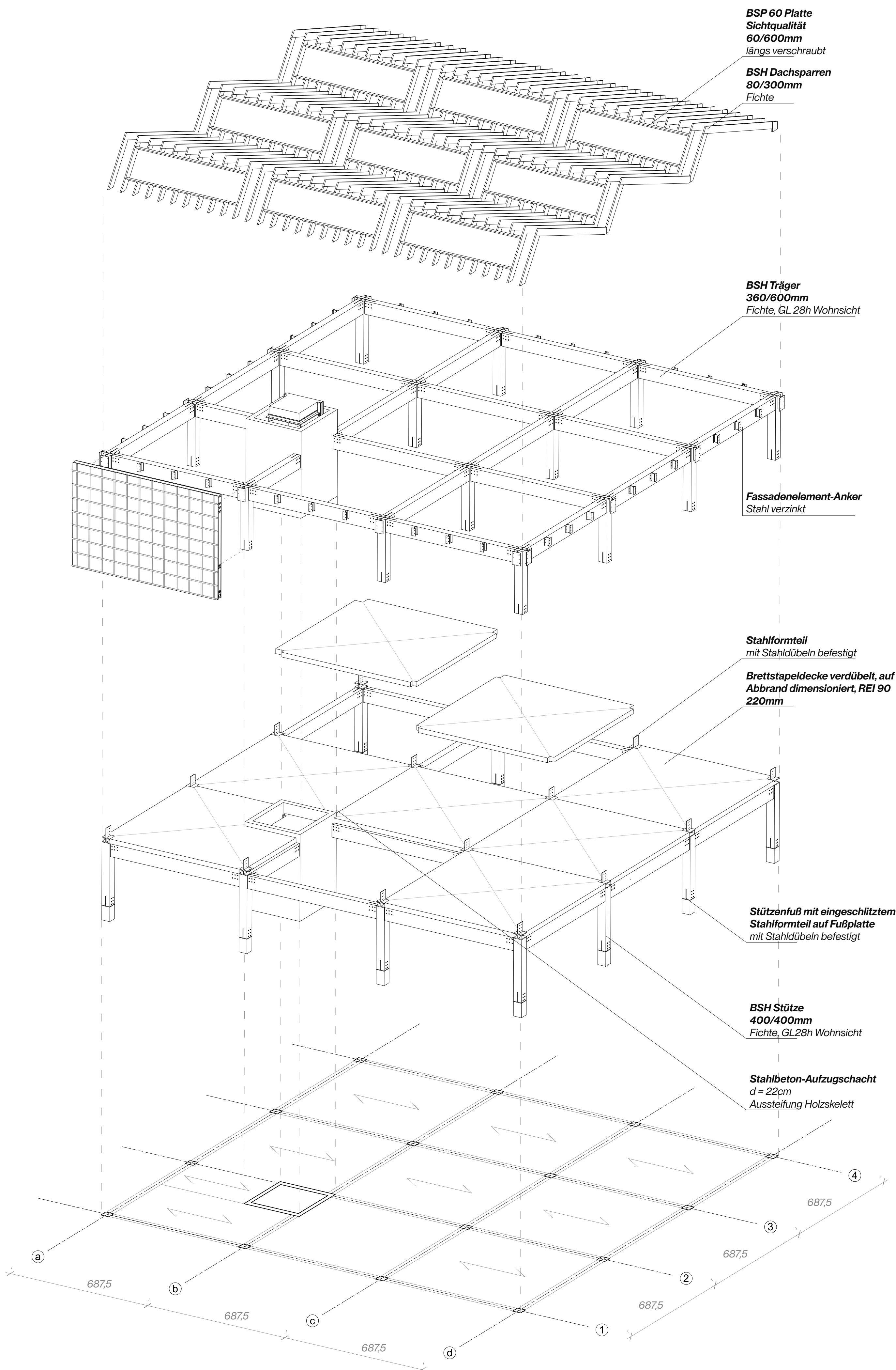
Tragwerksaxonomie Kindertagesstätte
