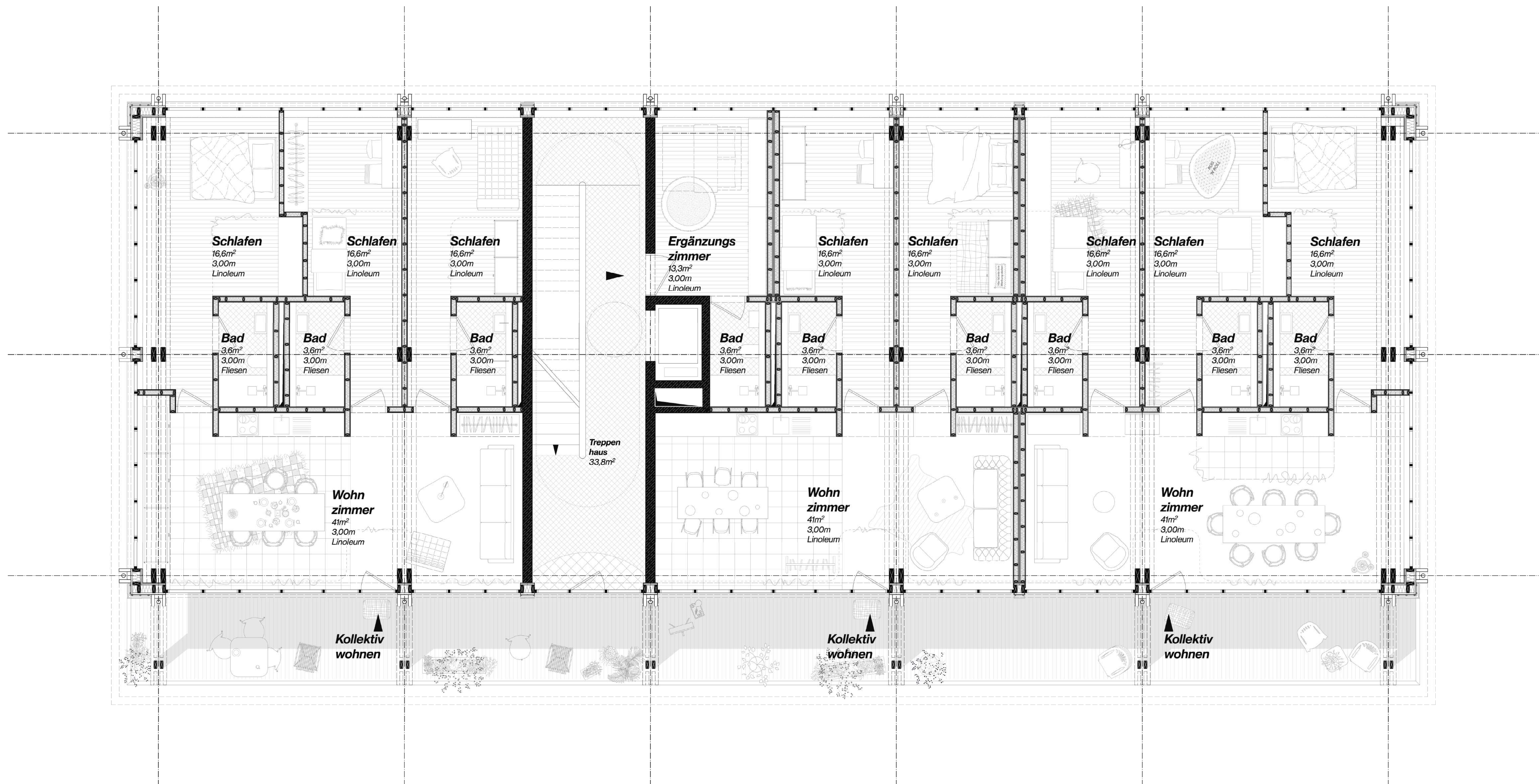
Grundriss 2. Obergeschoss 1:50
