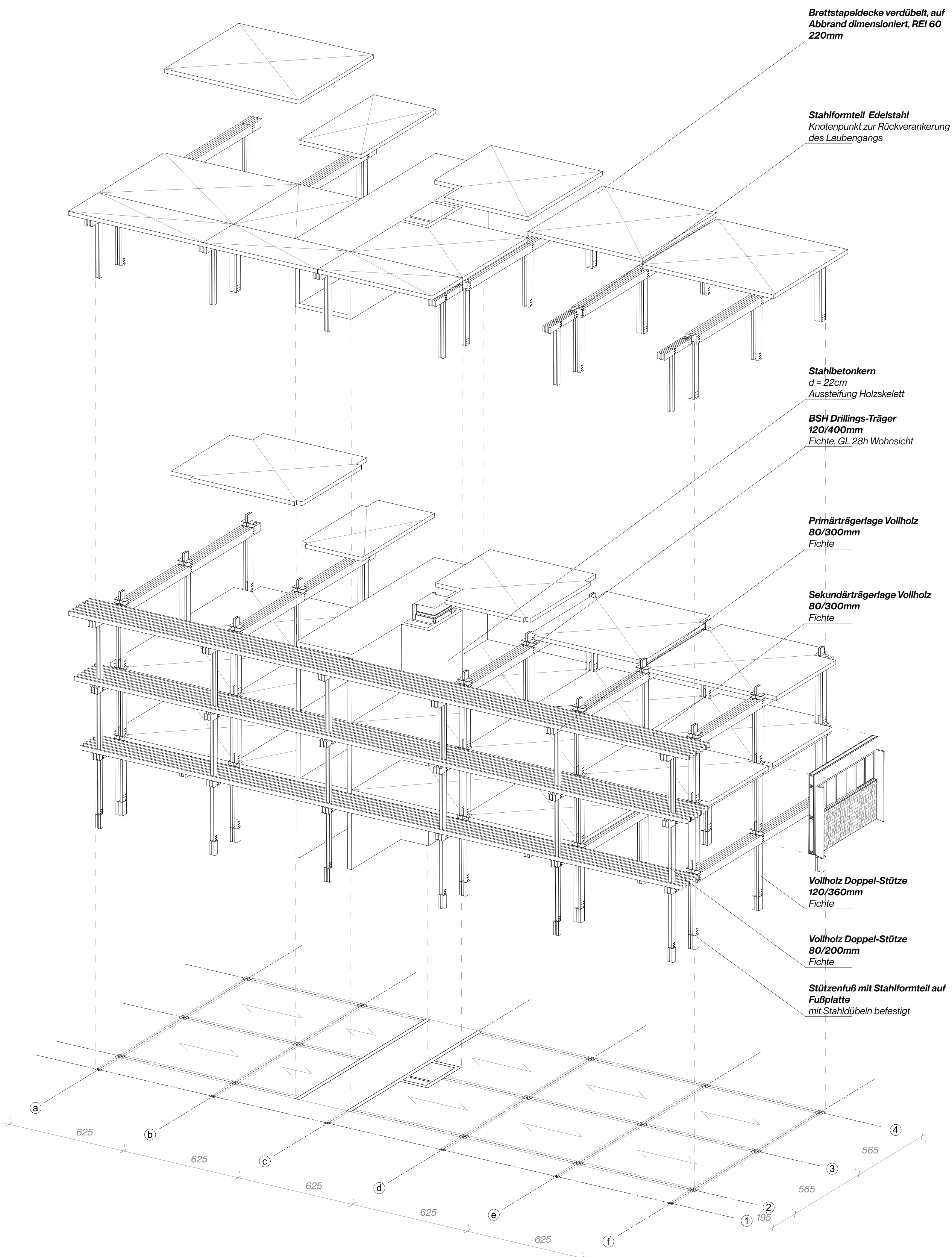
Tragwerksaxonomie Werkhaus
