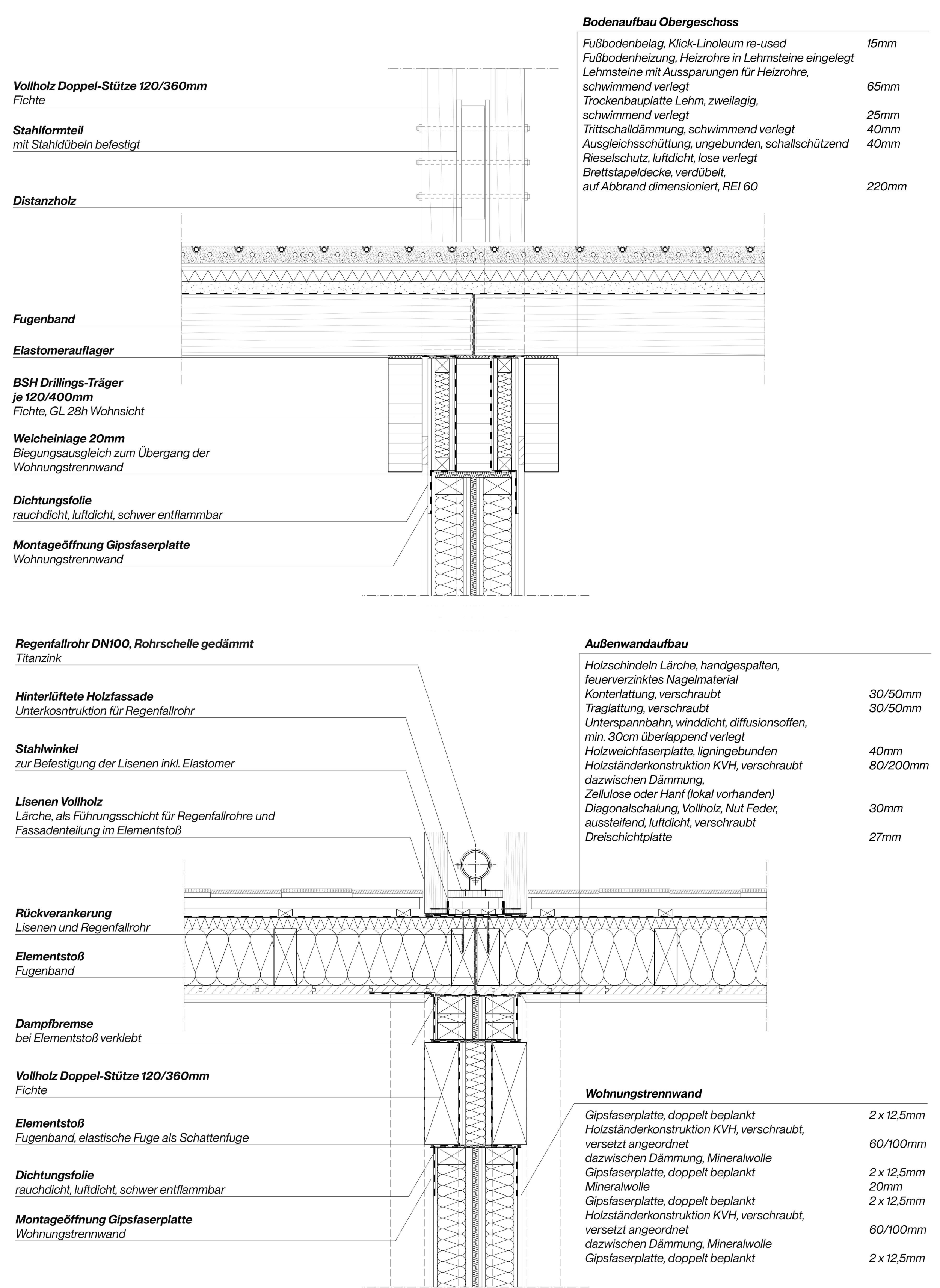
Detail Wohnungstrennwand 1:10
