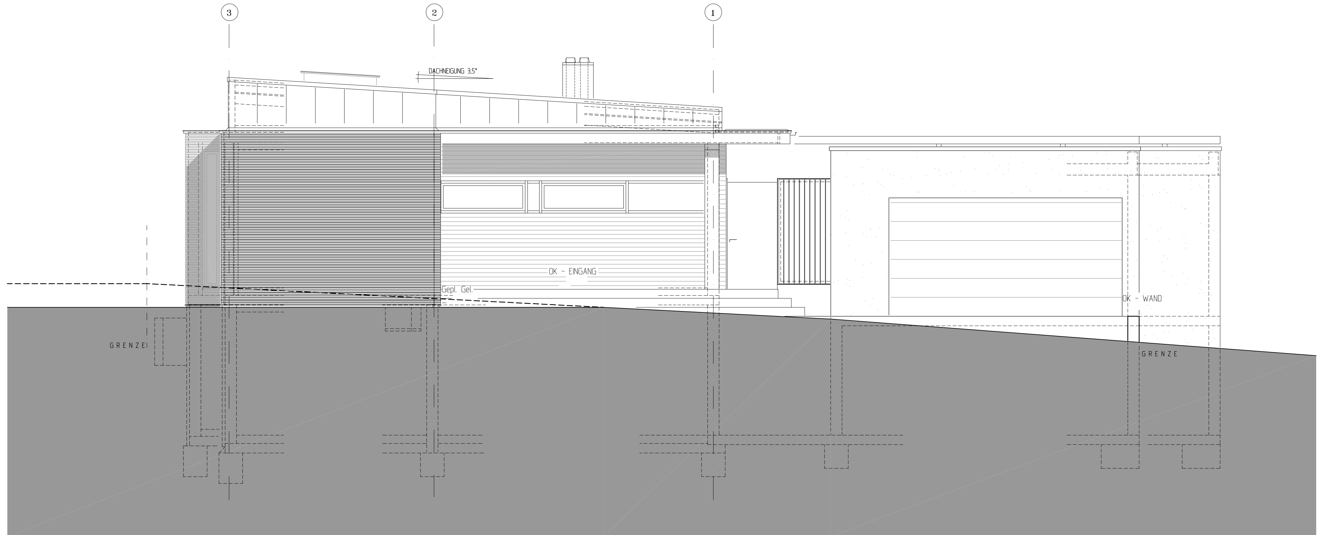
ANSICHT - WEST
