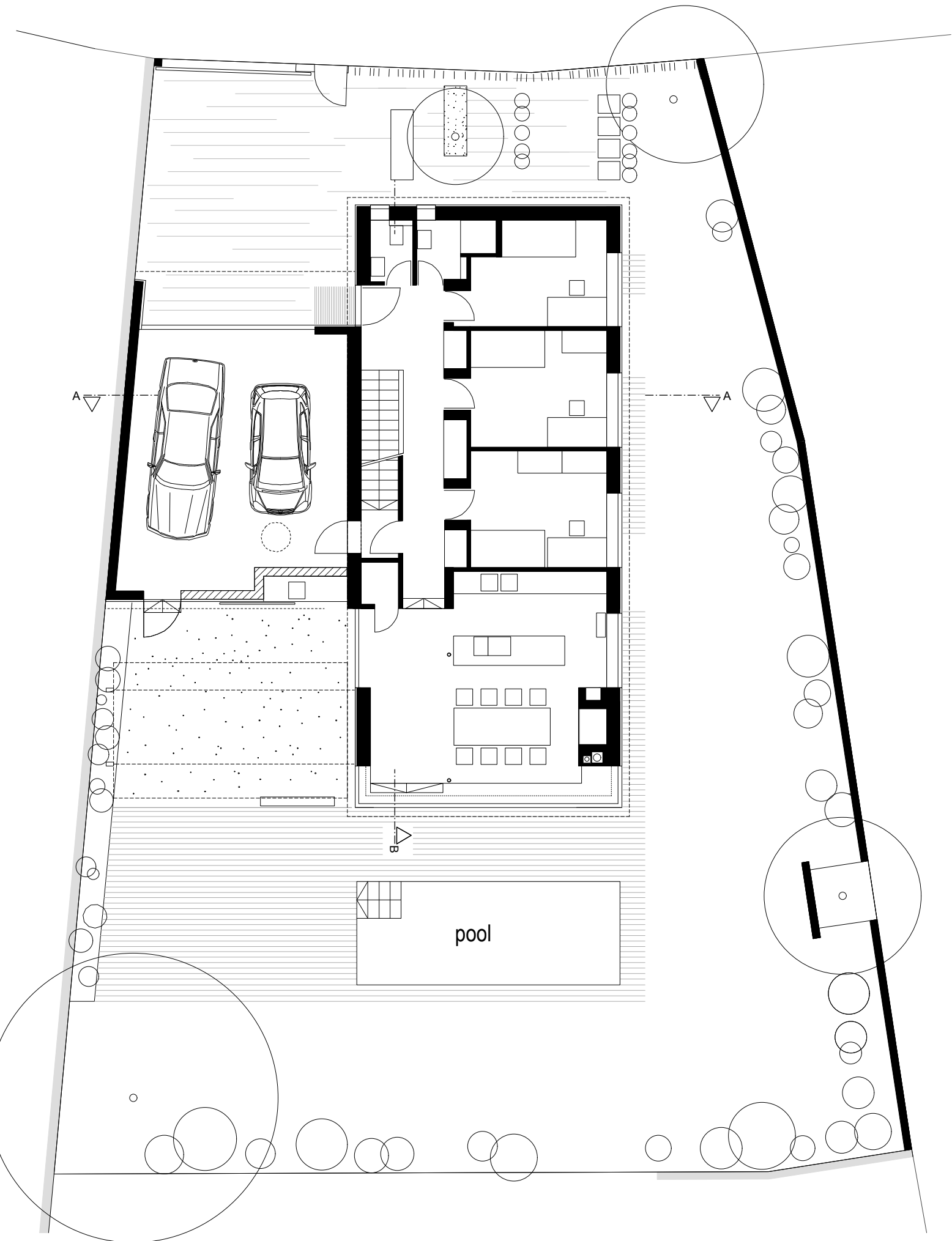
grundriss eg
