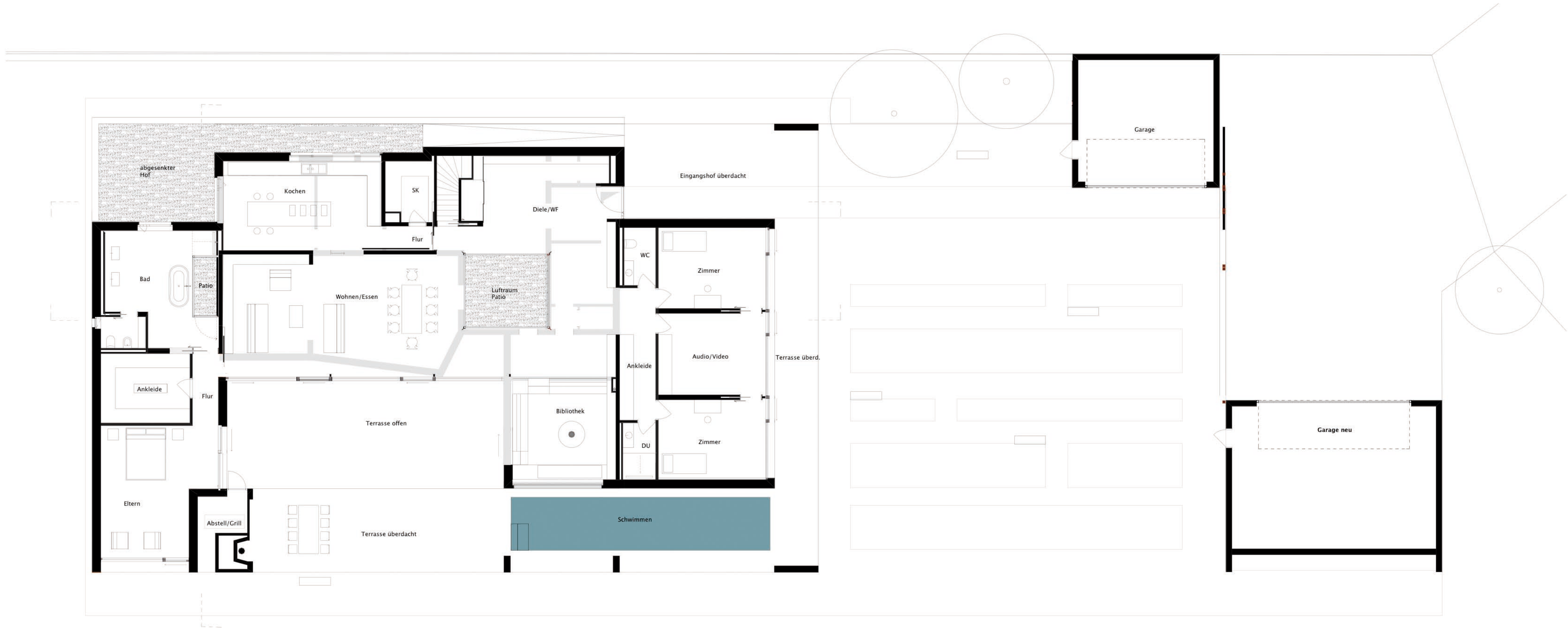
Grundriss Erdgeschoß M 1:125
