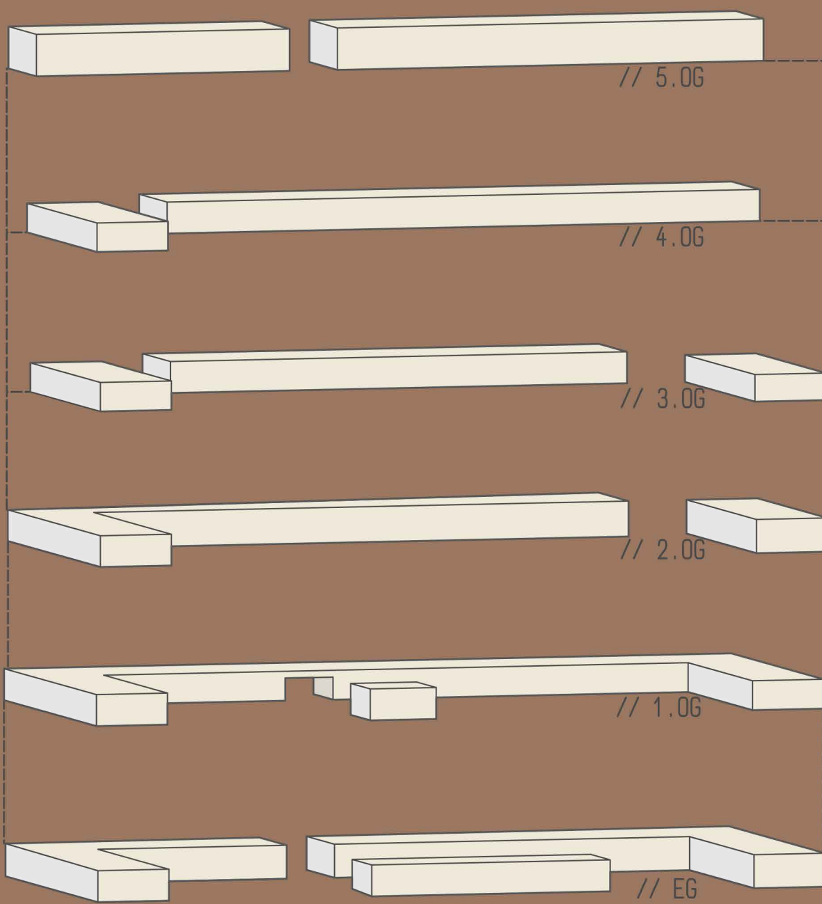
_staffelung der einzelnen geschossebenen
