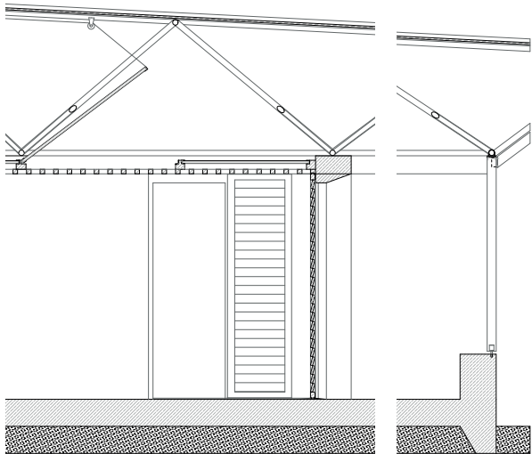
Detailschnitt Vertikal M 1:20
