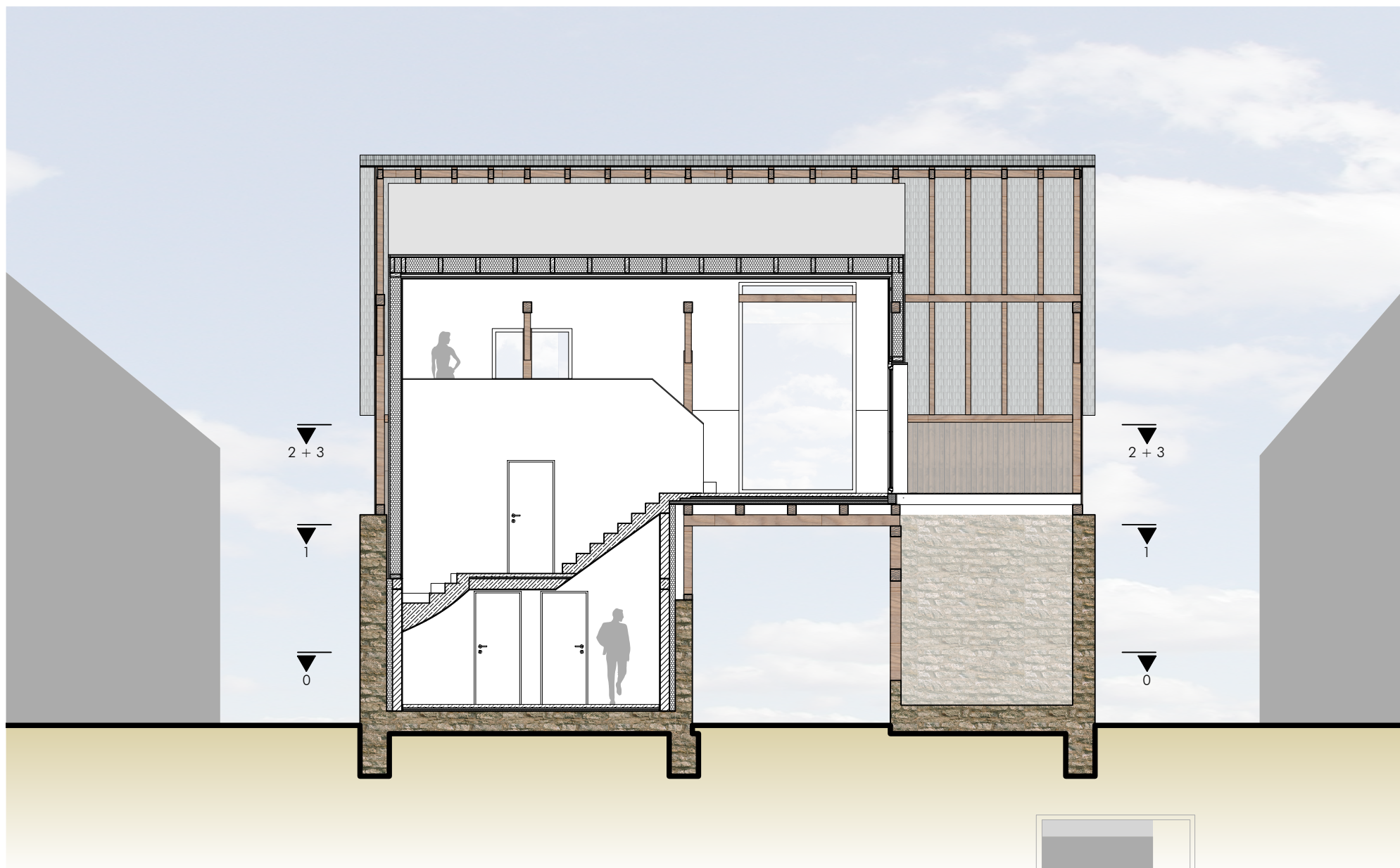
SCHNITT E-E
