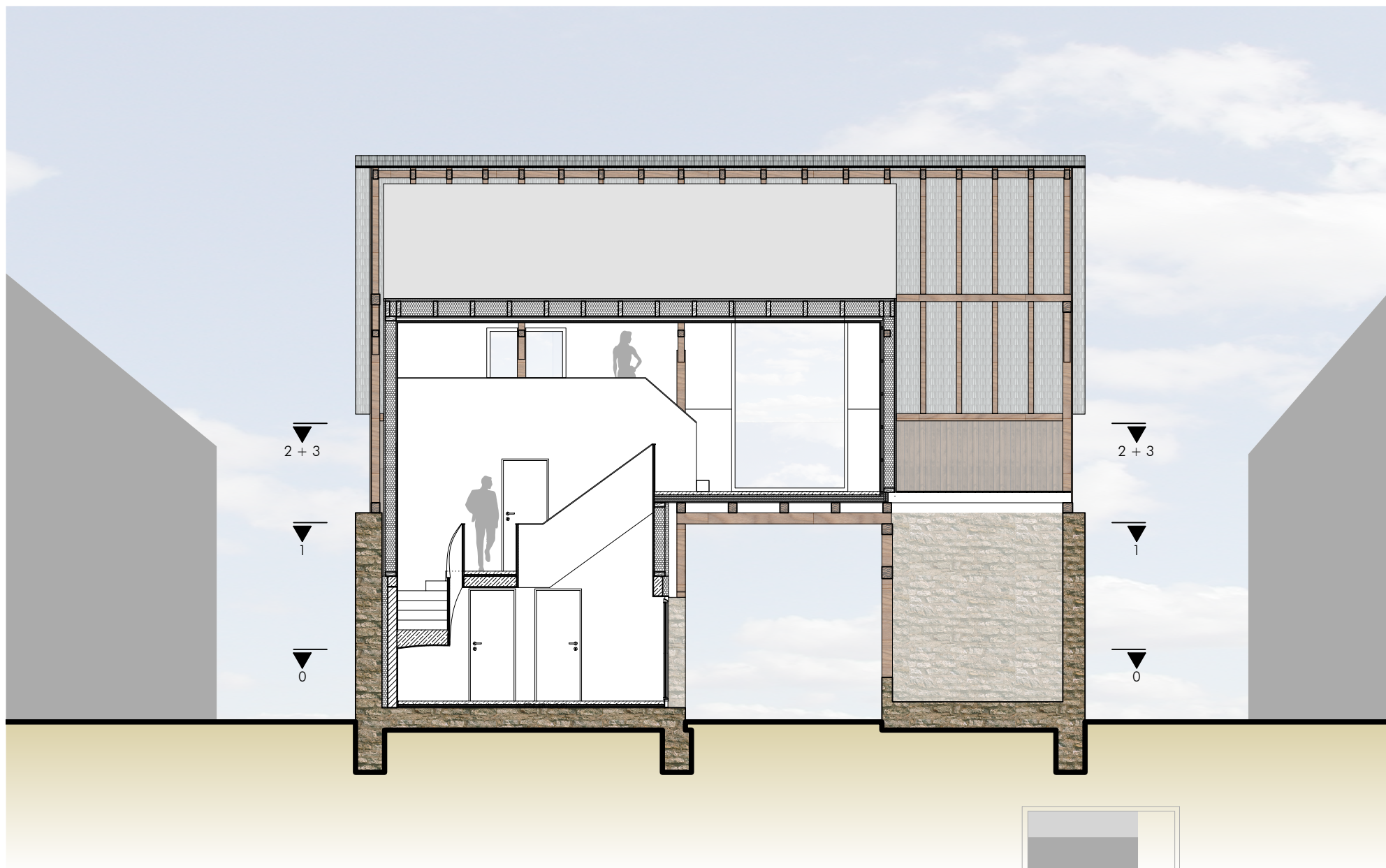
SCHNITT F-F
