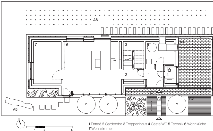
GRUNDRISS EG
