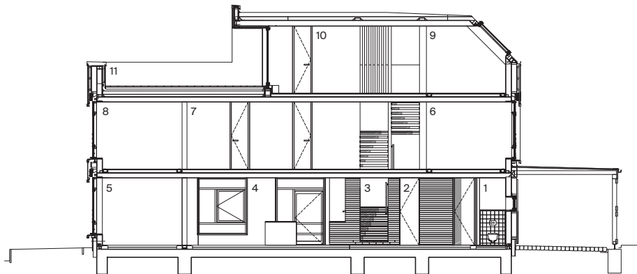
1 Gäste-WC 2 Flur 3 Treppenhaus 4 Wohnküche 5 Zimmer 6 Zimmer 7 Sonnendiele 8 Zimmer 9 Dachzimmer 10 Flur 11 Dachterrasse
