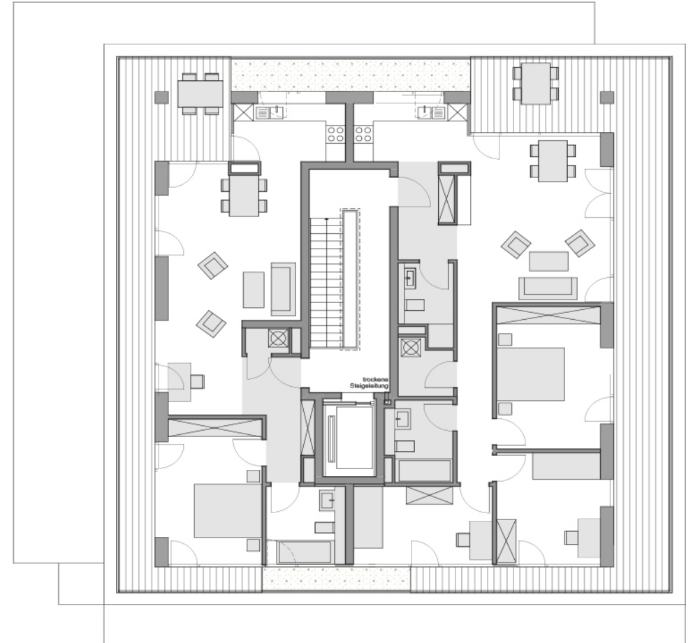
GR Dachgeschoss
