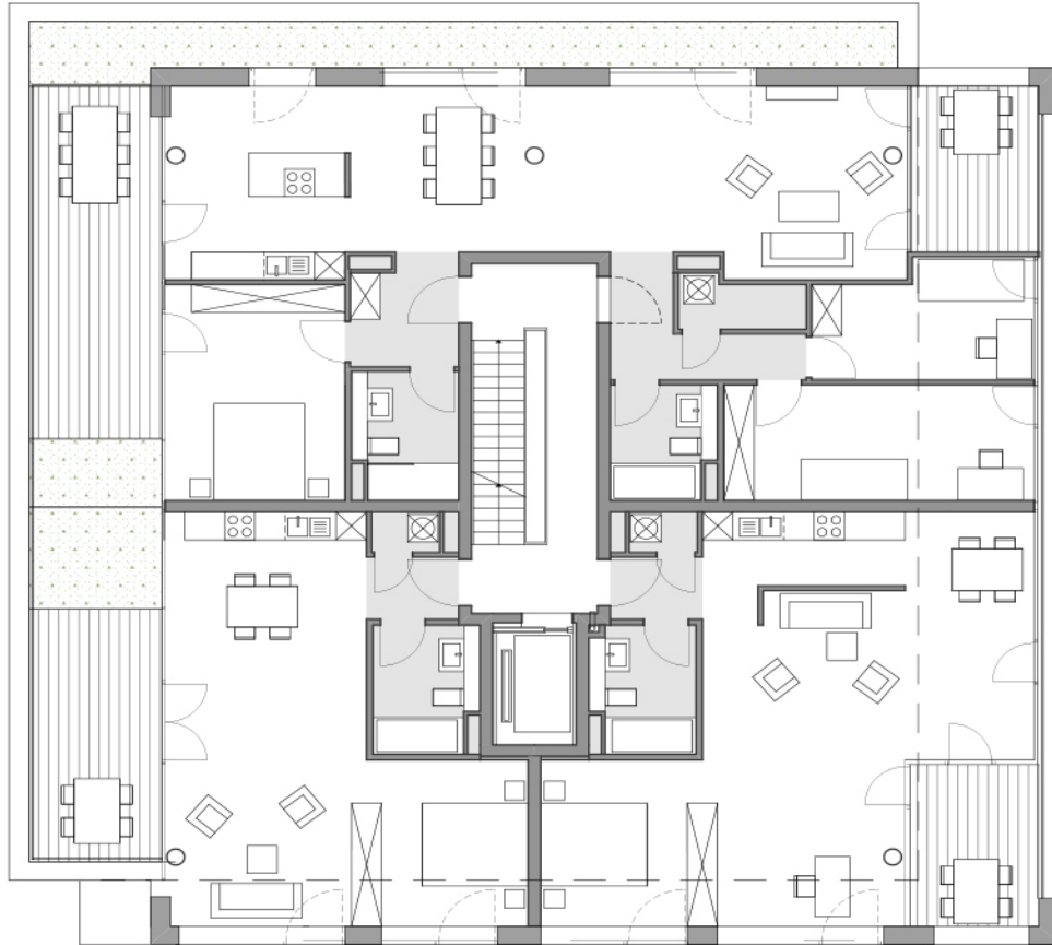
GR 4.Obergeschoss
