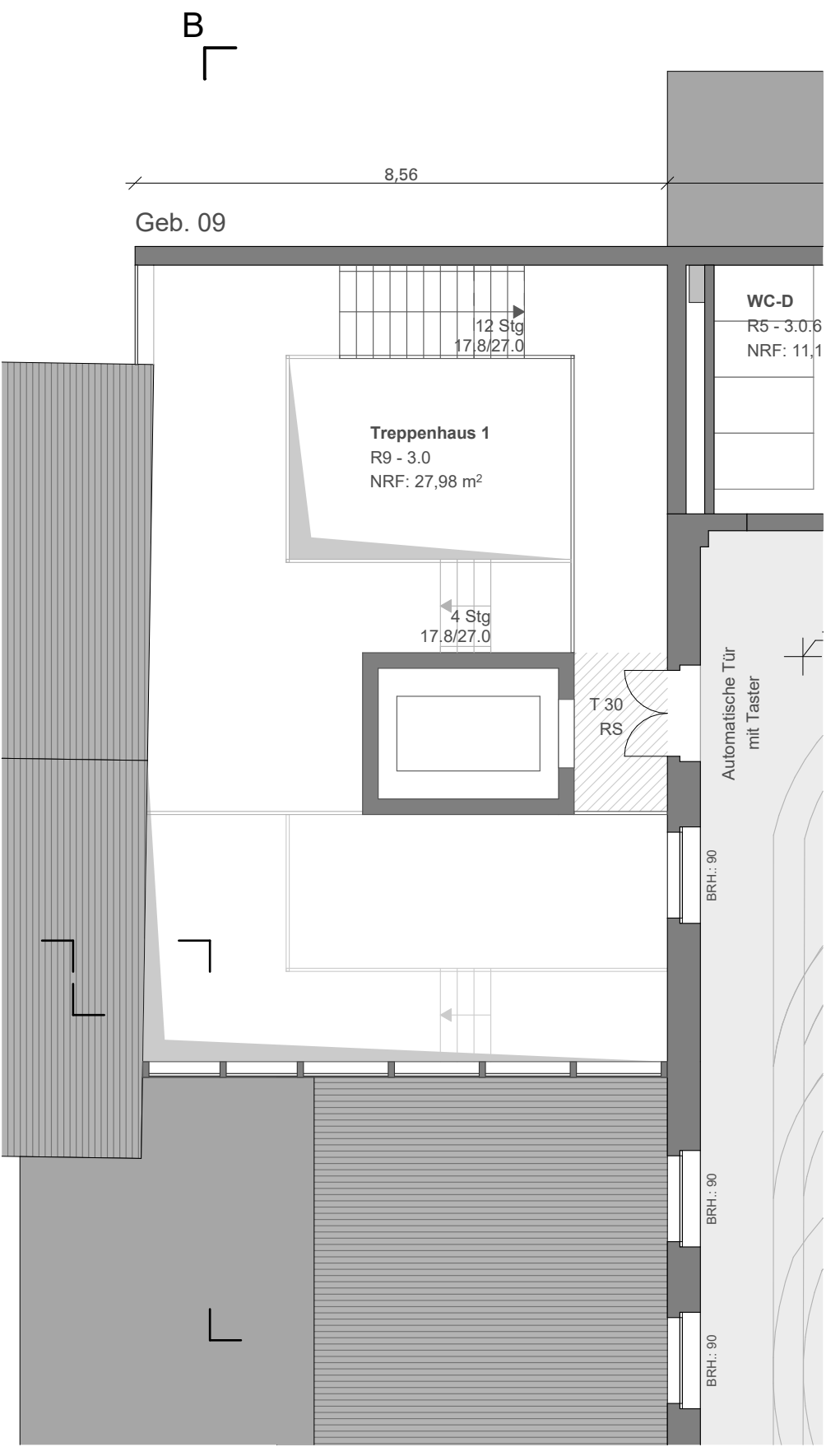
Grundriss 2.Obergeschoss
