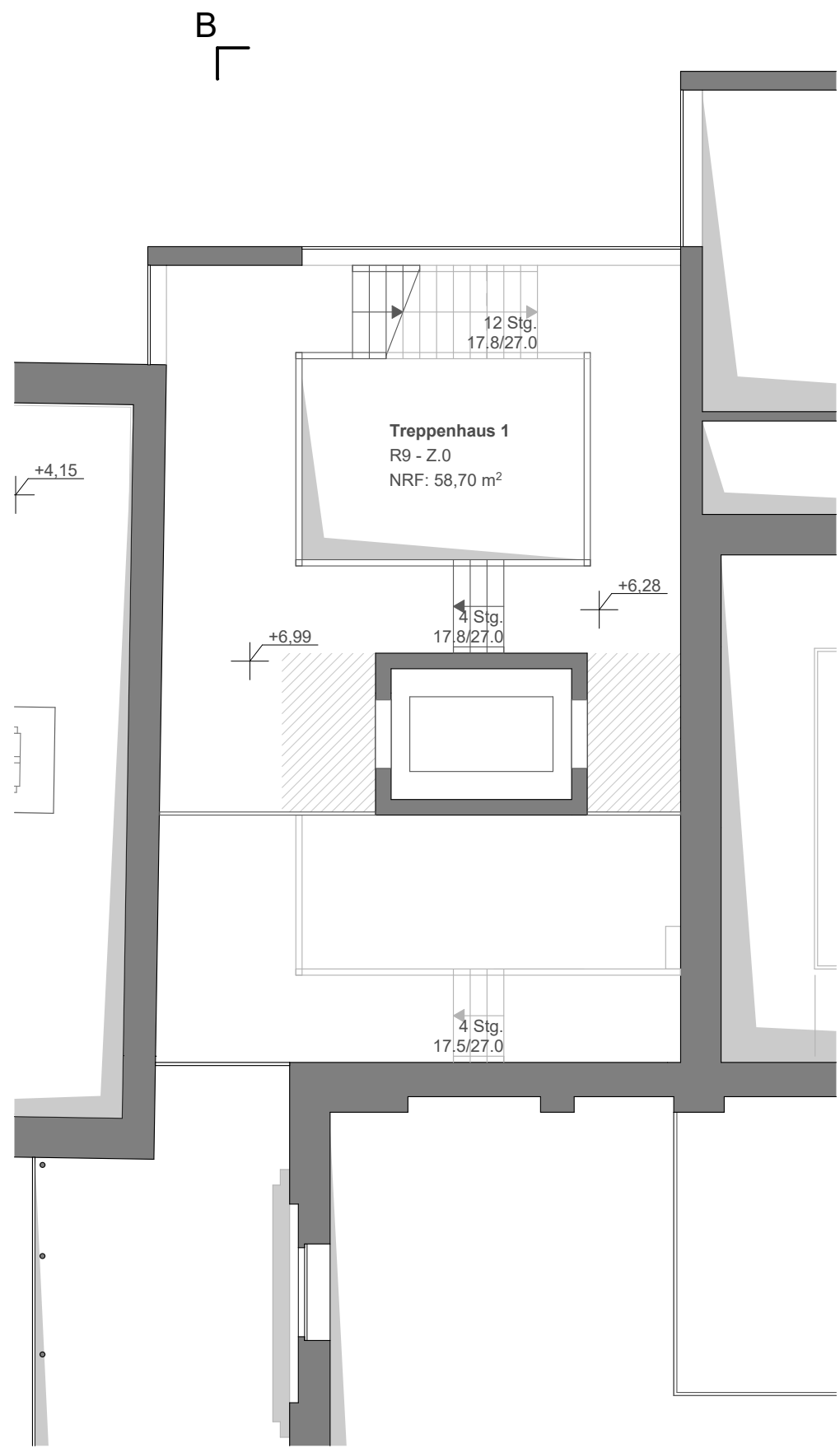
Grundriss Zwischengeschoss
