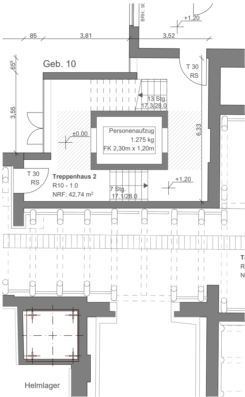
Grundriss Erdgeschoss
