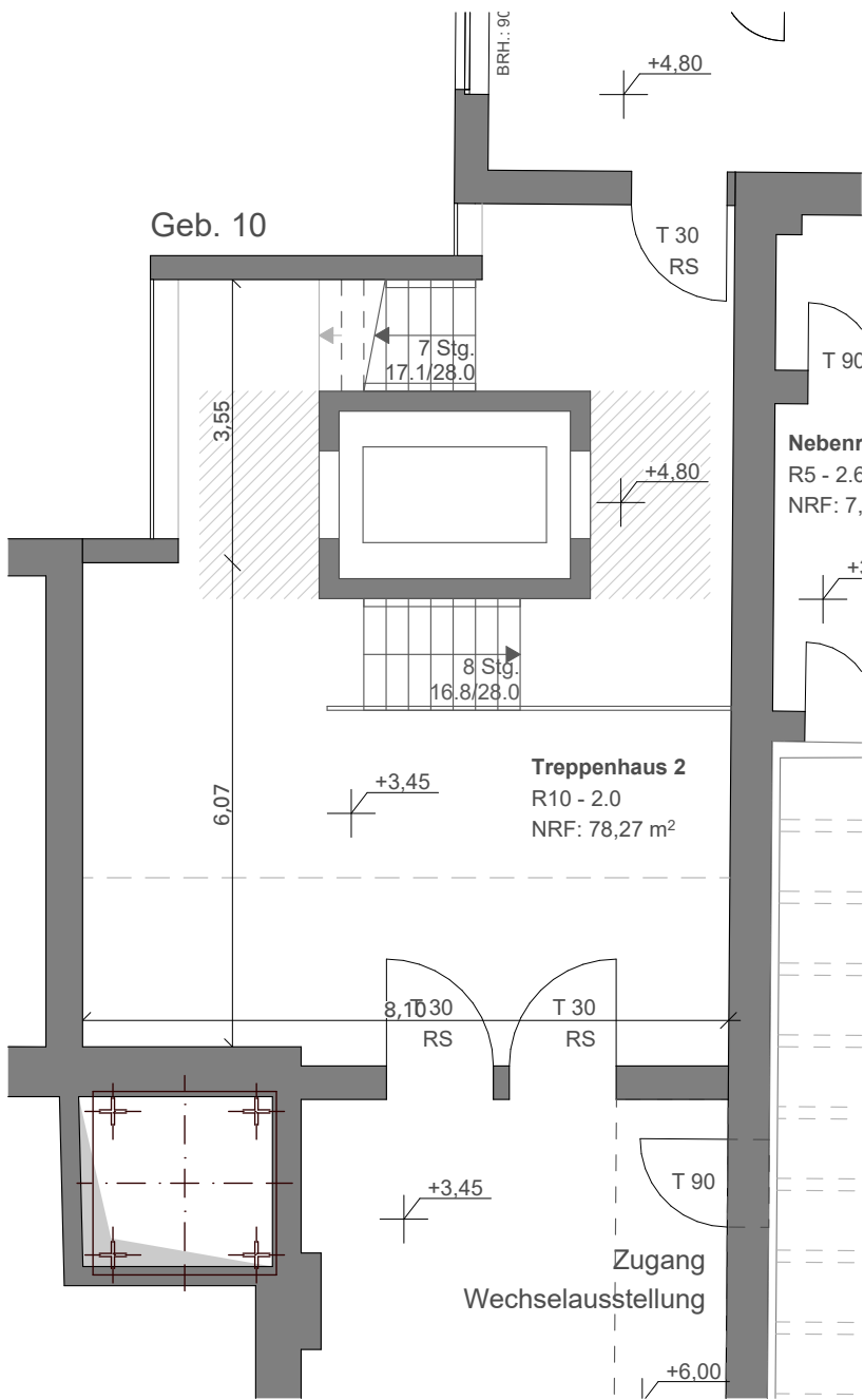
Grundriss 1. Obergeschoss
