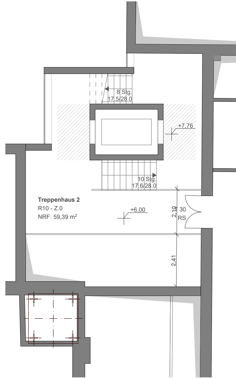
Grundriss Zwischengeschoss
