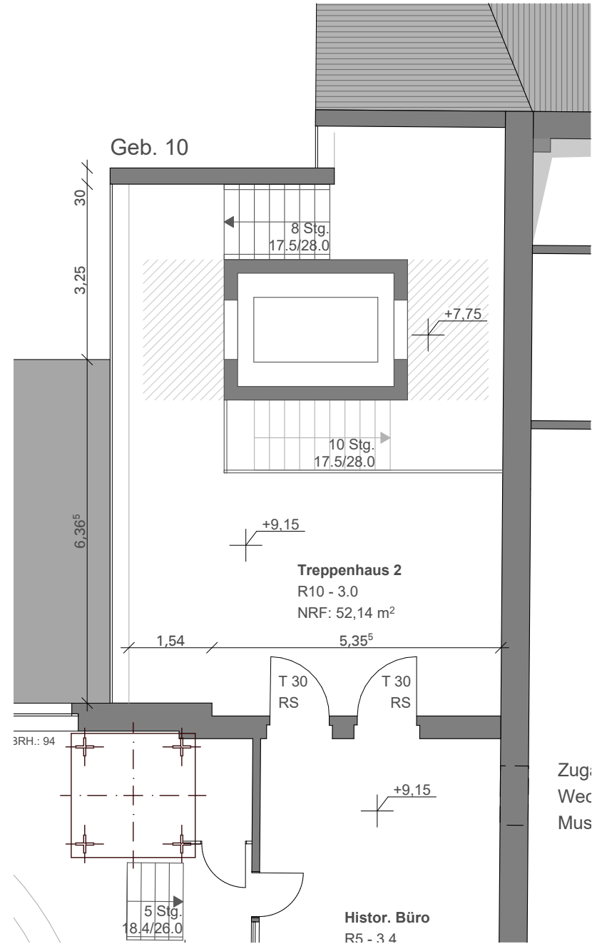
Grundriss 2.Obergeschoss
