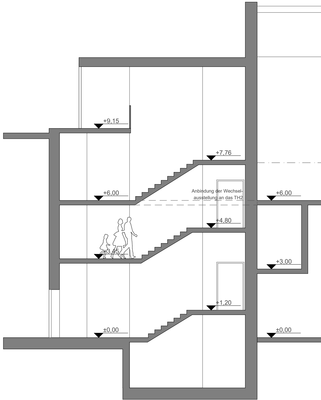
Schnitt D-D Treppenhaus 2
