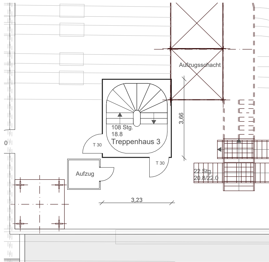
Grundriss 2.Obergeschoss
