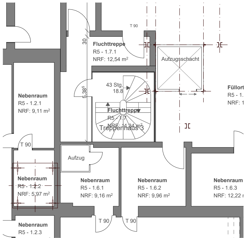
Grundriss Erdgeschoss
