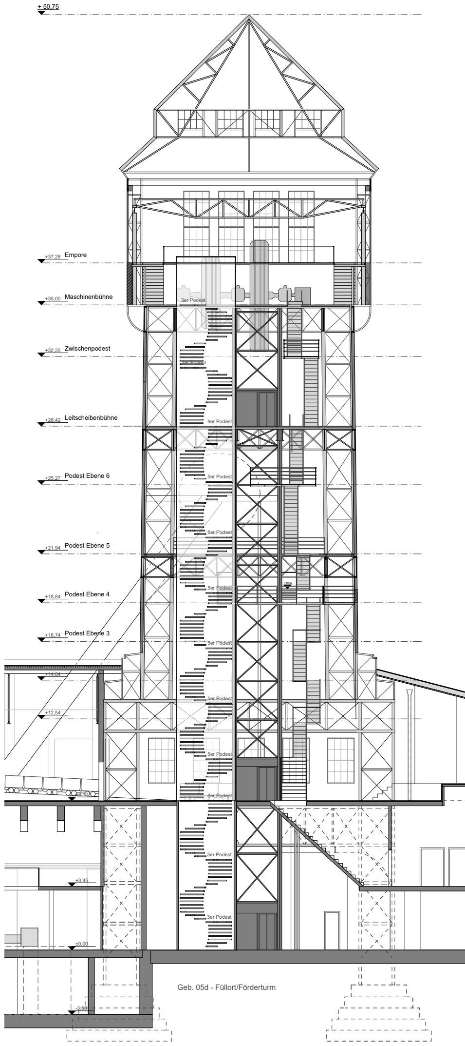
Ausschnitt Gesamtschnitt A-A Fluchttreppe
