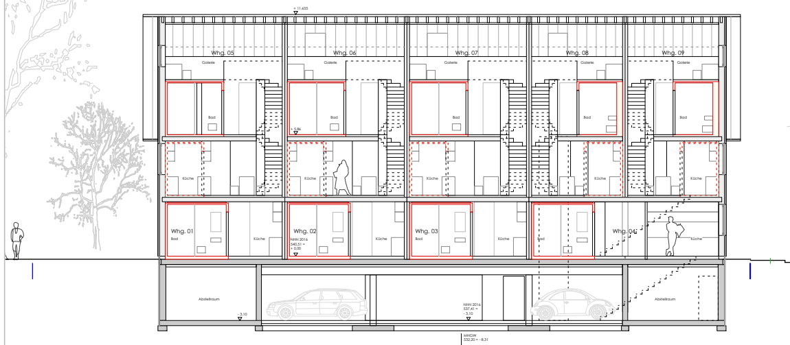
Schnitt Längs m = 1 | 250
