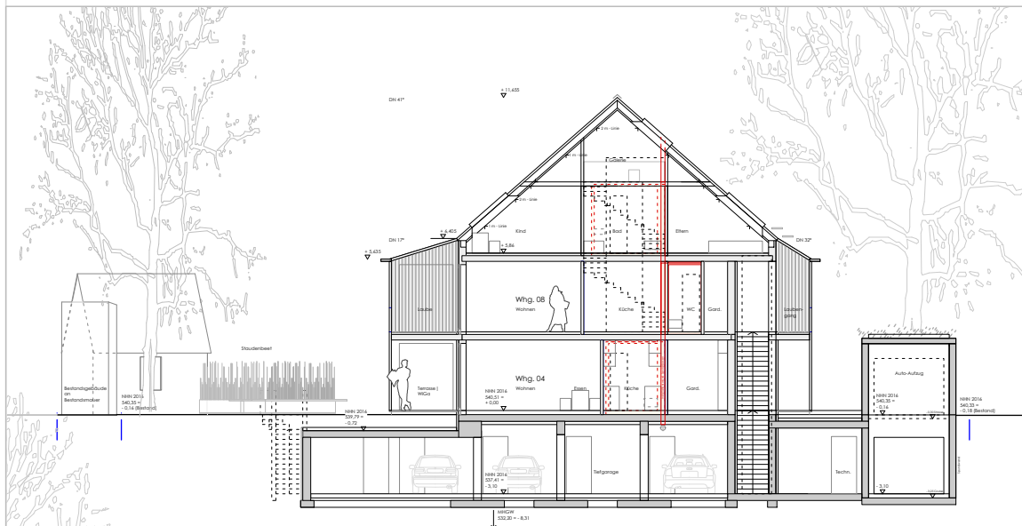
Schnitt Quer m = 1 | 250
