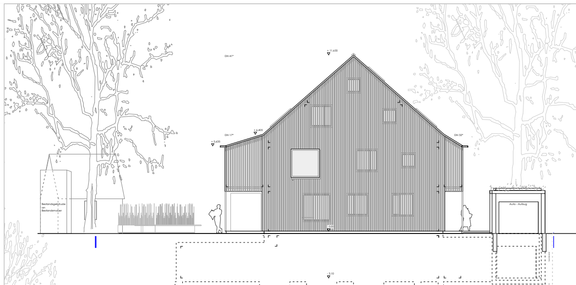
Ansicht Osten m = 1 | 250
