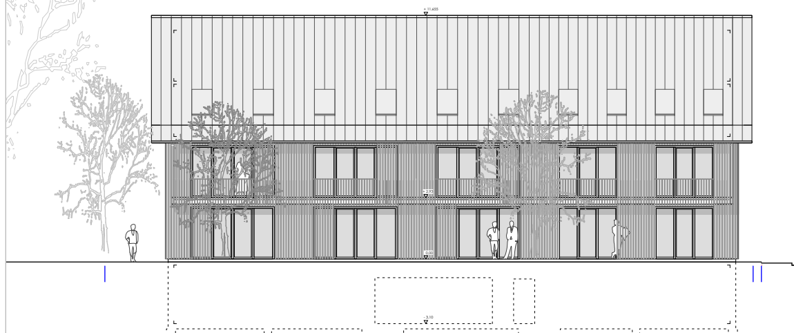
Ansicht Osten m = 1 | 250
