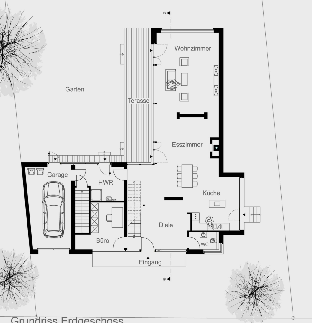
Grundriss Erdgeschoss
